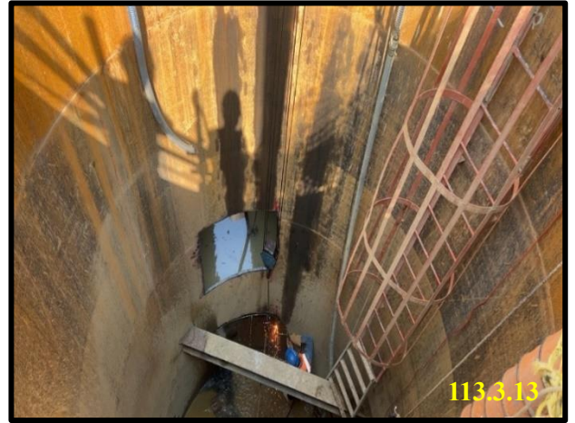
大潭北路到達井鋼環開孔
