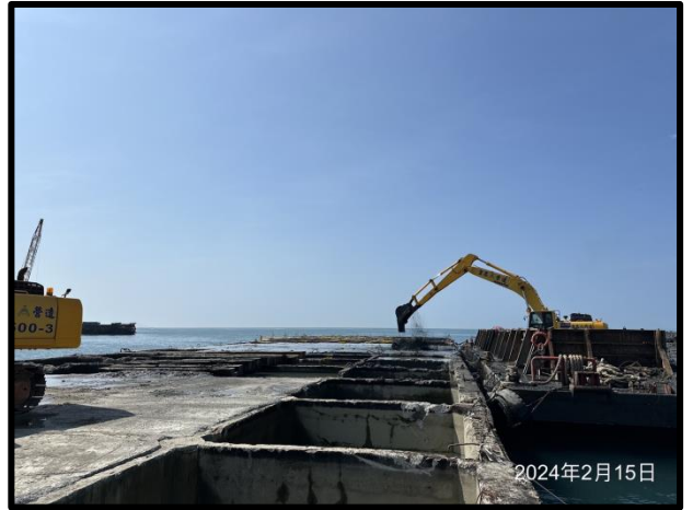
沉箱(#58~#59)回填砂作業
