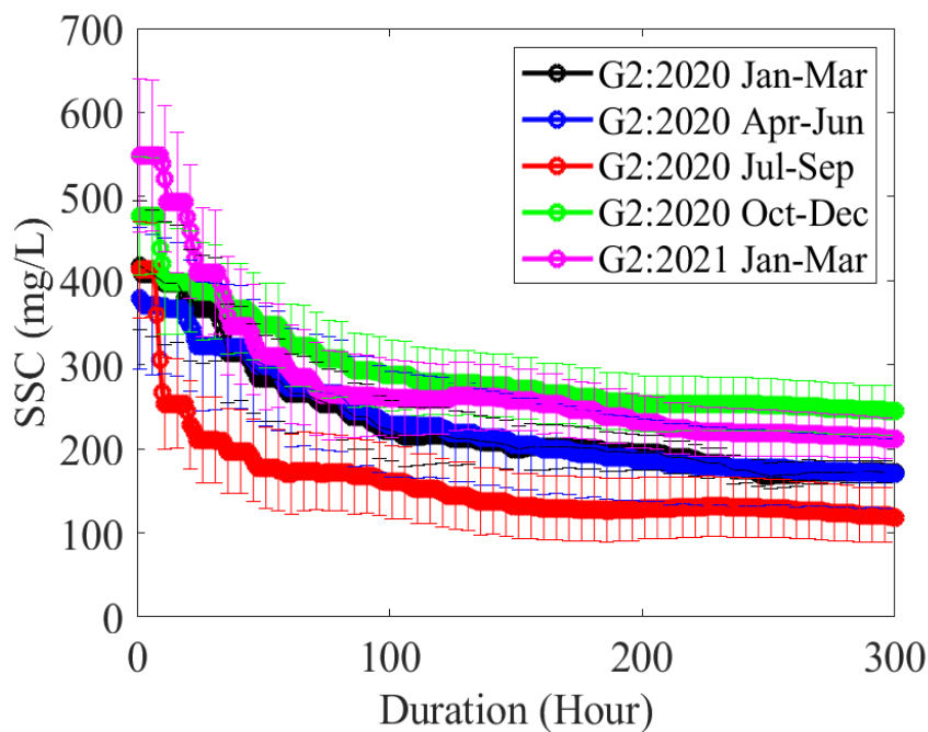
圖 3.1.12-1 G2 區懸浮漂沙濃度 110 年第 1 季與歷次逐時監測值比對圖
