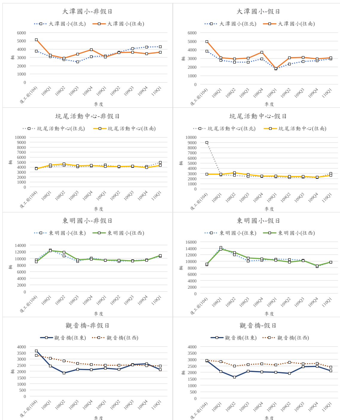
圖 3.1.6-1 歷次路段交通量監測結果分析圖
