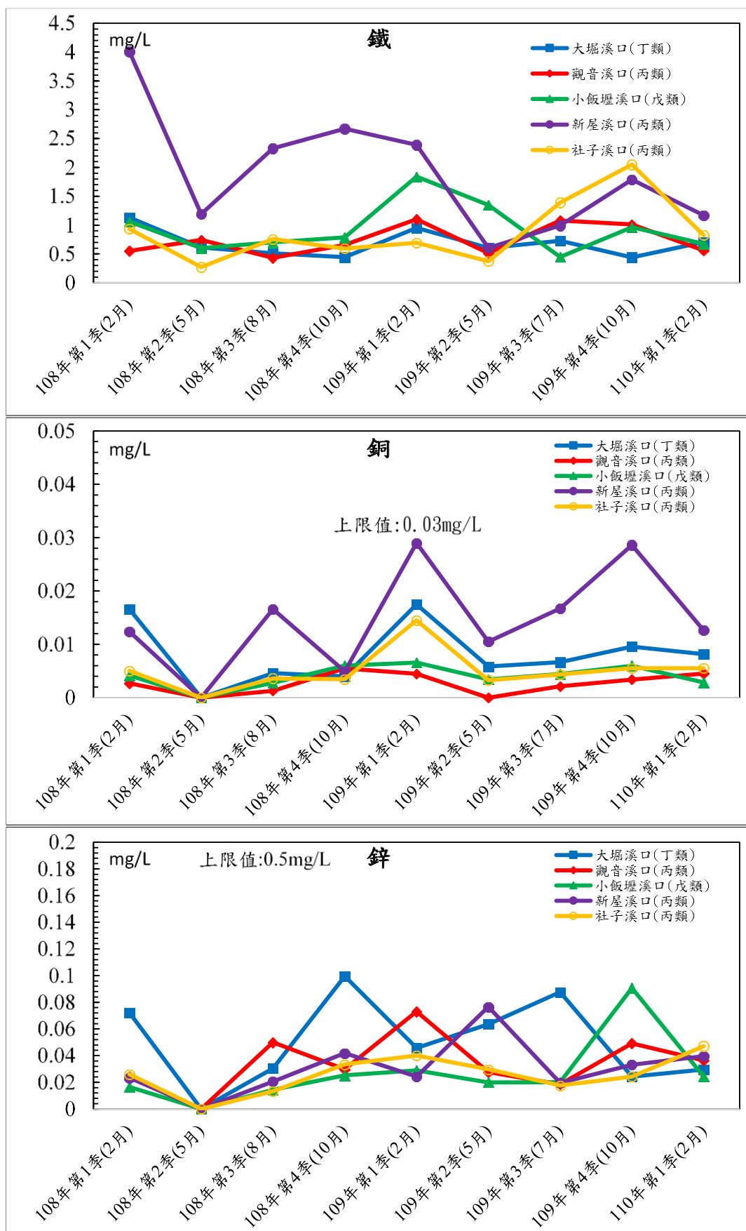
圖 3.1.7-1 歷次河口水質監測結果分析圖(6/8)
