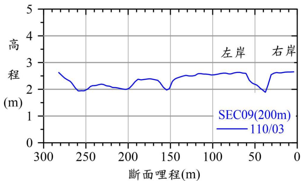
圖 2.12.1-8 觀音溪河口地形斷面圖(SEC07~SEC09)
