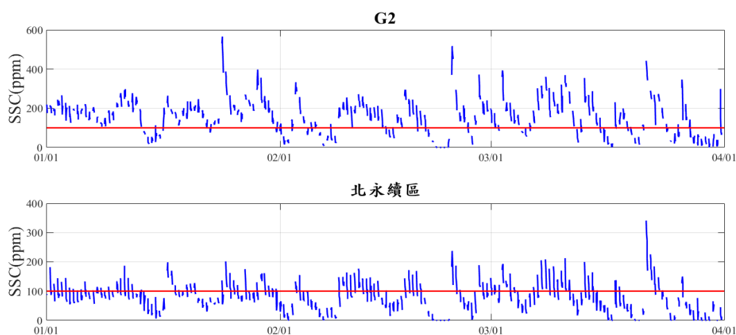
圖 2.11.1-2 漂沙濃度逐時資料時序列圖
