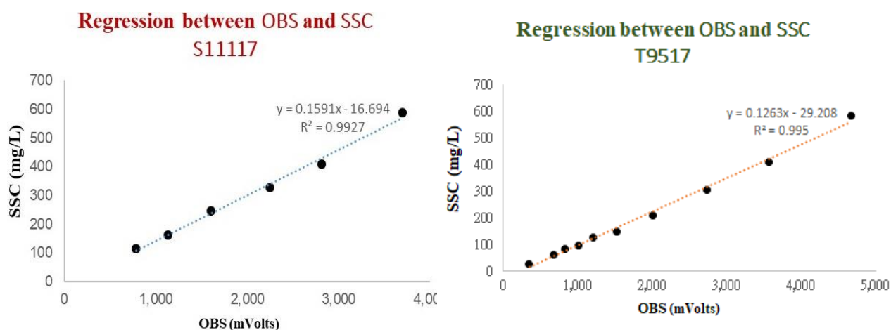
圖 1.8.1-1 光學濁度計率定結果圖
