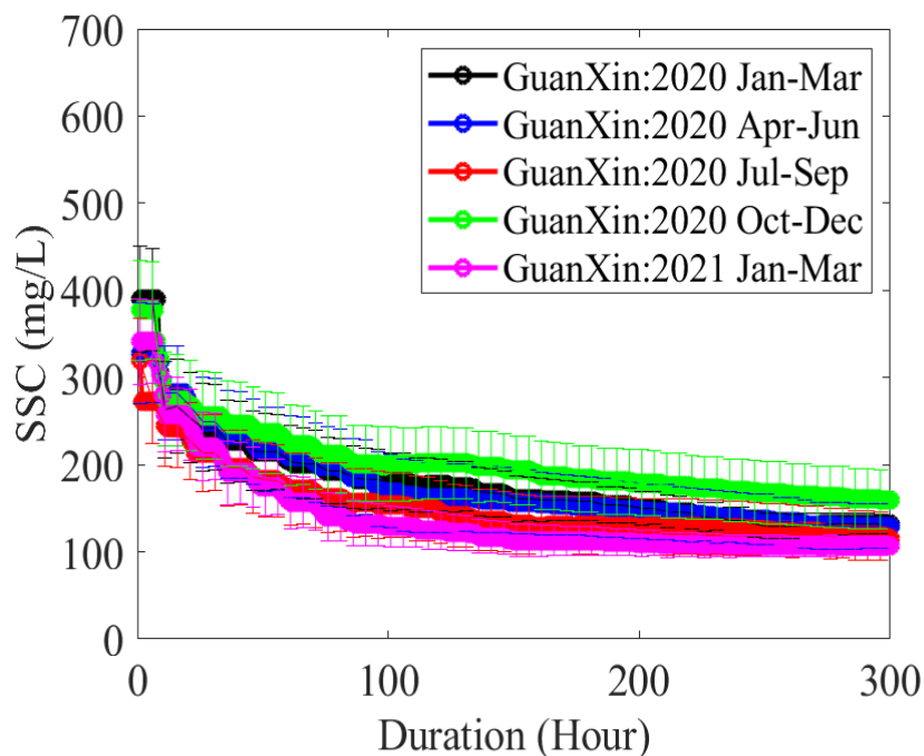
圖 3.1.12-2 保護區懸浮漂沙濃度 110 年第 1 季與歷次逐時監測值比對圖
