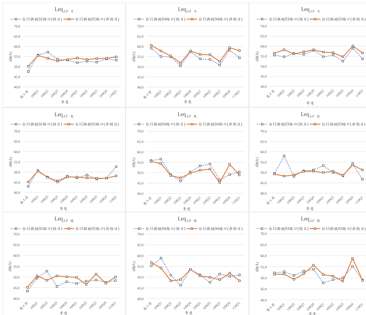
圖 3.1.5-1 歷次低頻噪音監測結果分析圖
