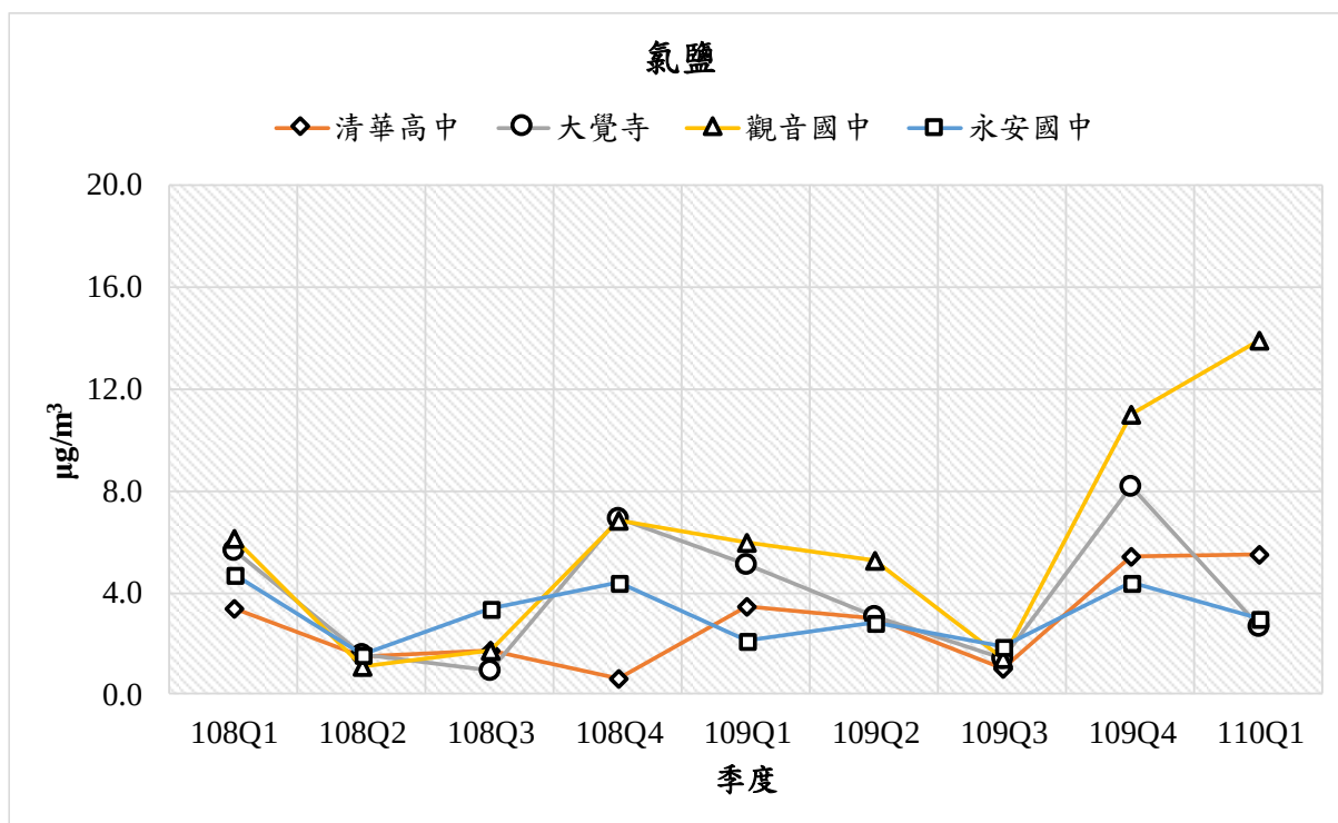
圖 3.1.2-12 鹽份監測結果分析圖
