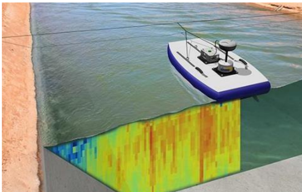
圖 1.8.2-4 船攜 ADCP 走航量測示意圖
