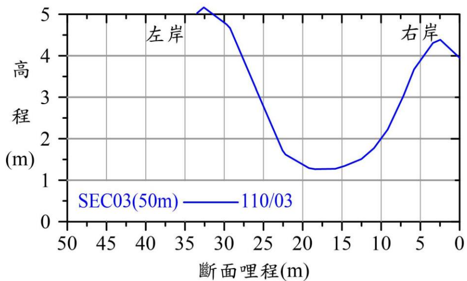
圖 2.12.1-6 觀音溪河口地形斷面圖(SEC01~SEC03)
