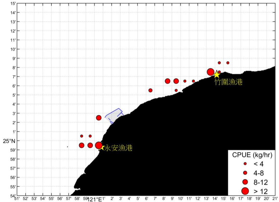
圖 2.10.2-8 109 年 12 月桃園地區每單位努力漁獲量(CPUE)分布
