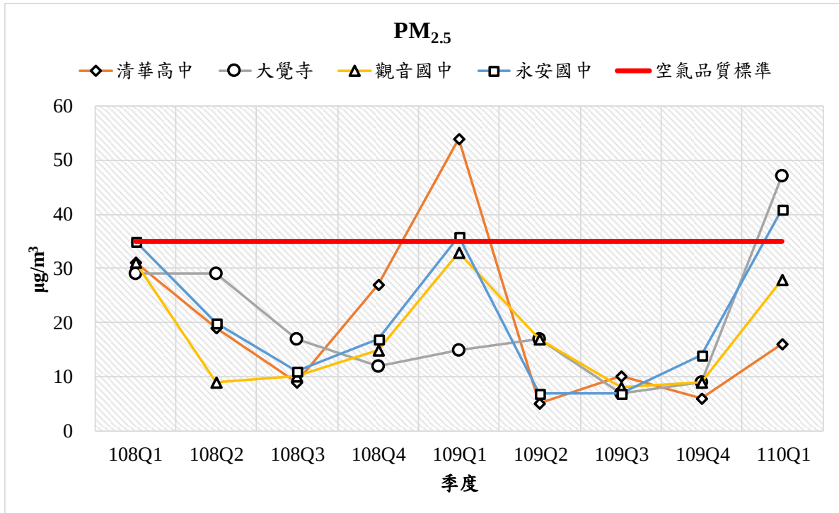
圖 3.1.2-3 PM 2.5 監測結果分析圖
