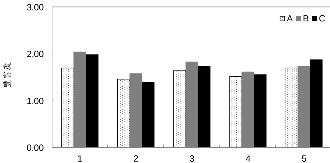
圖 2.8.2-3 110 年第 1 季海域各測站浮游動物大類數變化圖
