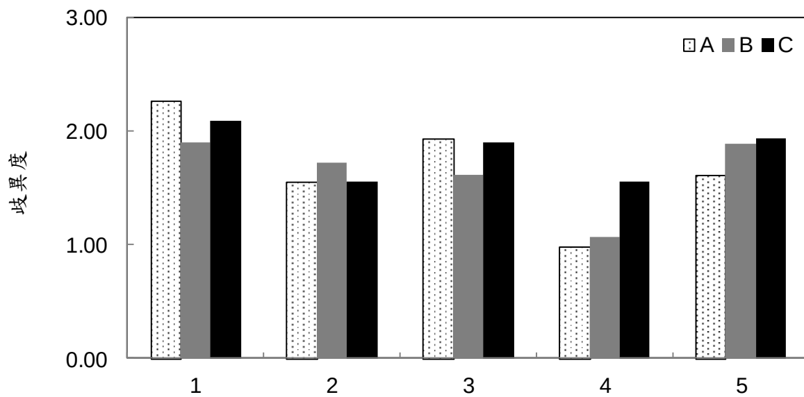
圖 2.8.2-5 110 年第 1 季海域各測站浮游動物均勻度變化圖
