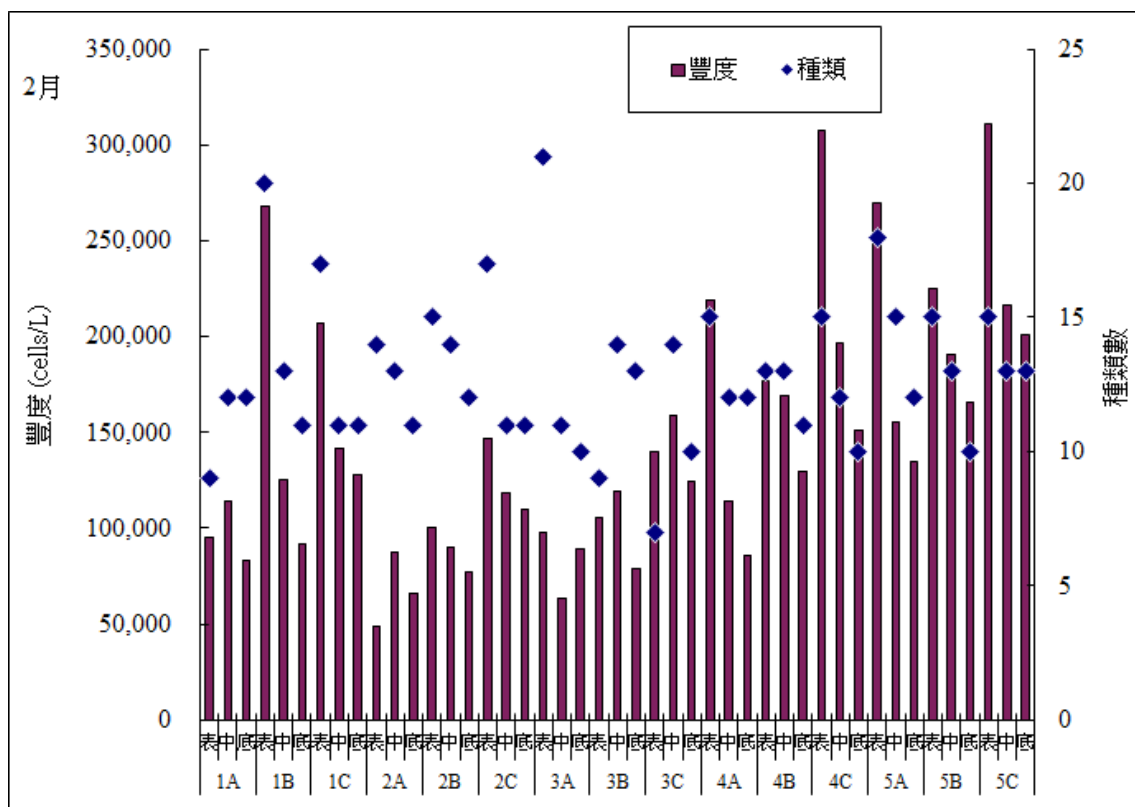
圖 2.8.1-1 110 年第 1 季海域各測站之浮游植物種類及數量分布圖
