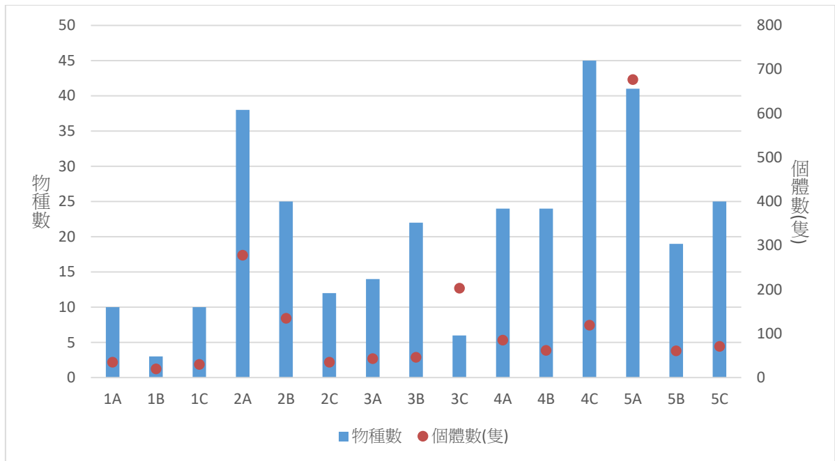
圖 2.8.3-1 110 年第 1 季海域各測站底棲生物之種類數及個體數比較圖
