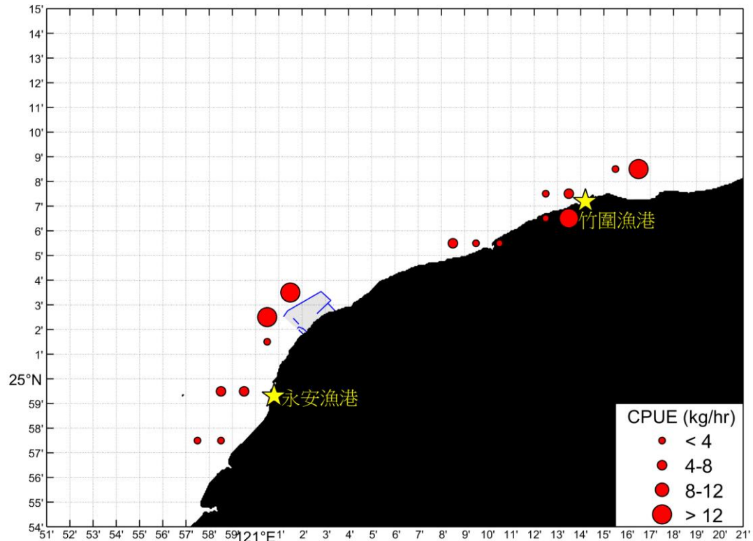
圖 2.10.2-10 110 年 2 月桃園地區每單位努力漁獲量(CPUE)分布
