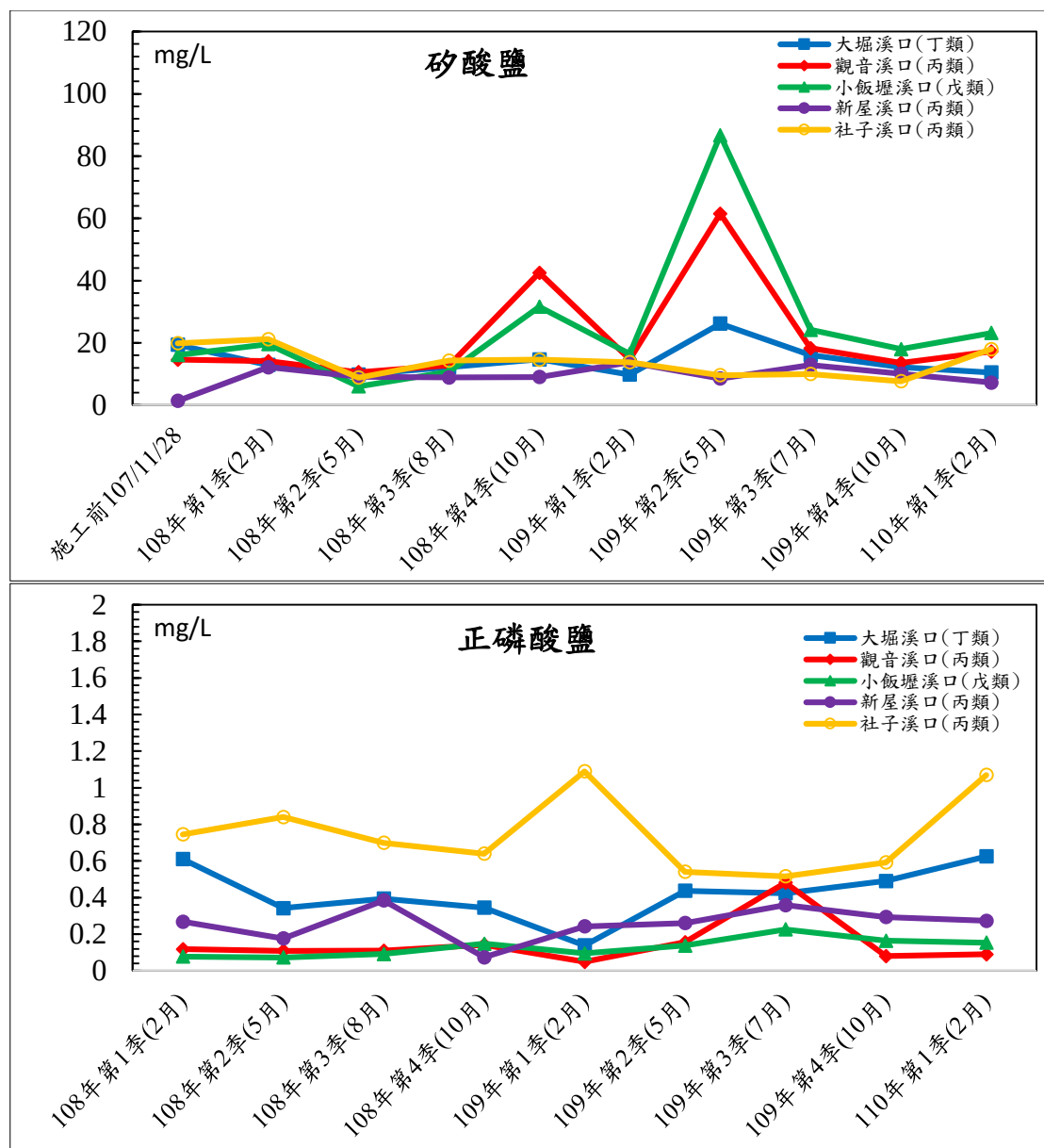
圖 3.1.7-1 歷次河口水質監測結果分析圖(8/8)
