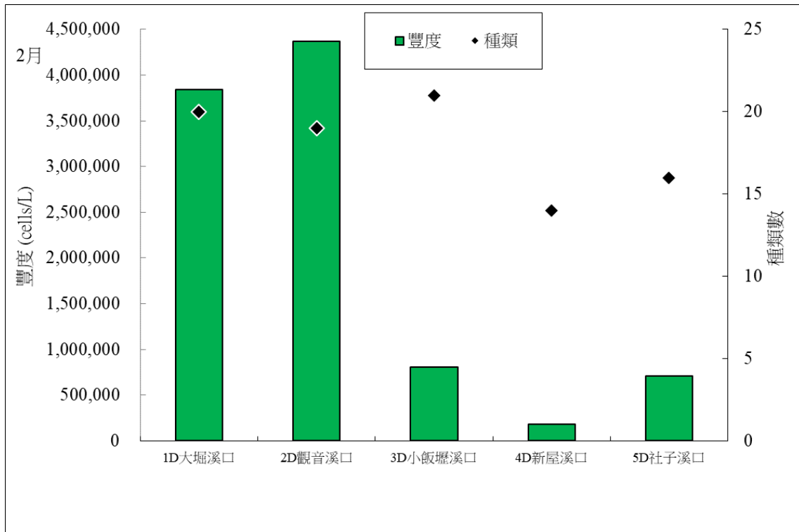
圖 2.9.1-1 110 年第 1 季河口各測站之浮游植物種類及數量分布圖
