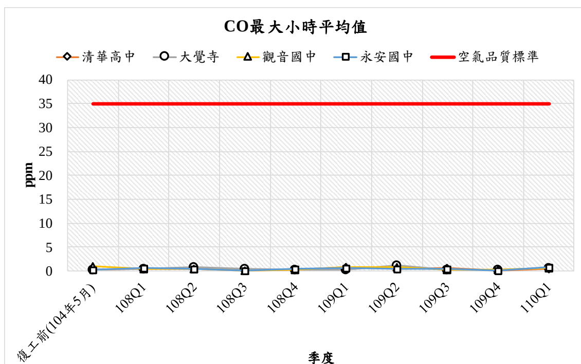
圖 3.1.2-8 CO 最大小時平均值監測結果分析圖
