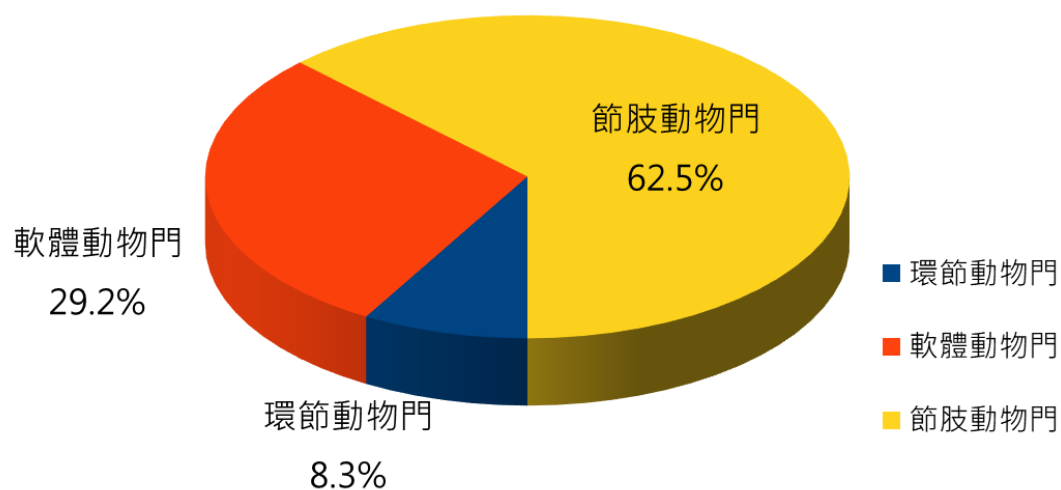
圖 2.9.3-3 110 年第 1 季河口各測站之底棲生物各大類個體數百分比
