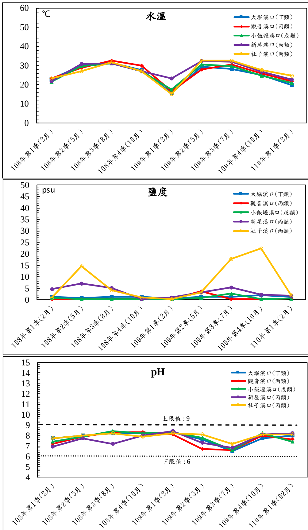
圖 3.1.7-1 歷次河口水質監測結果分析圖(1/8)
