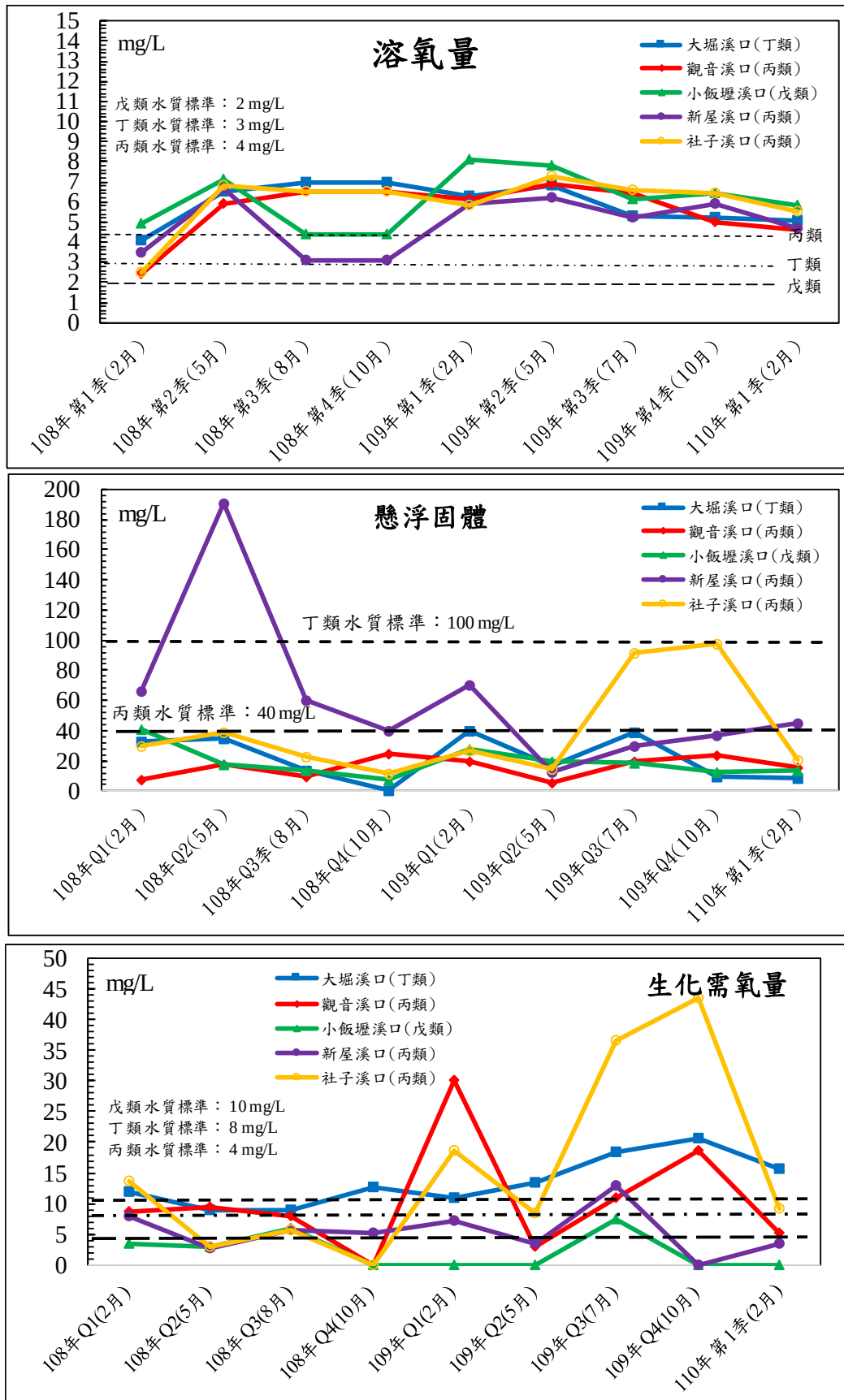
圖 3.1.7-1 歷次河口水質監測結果分析圖(2/8)
