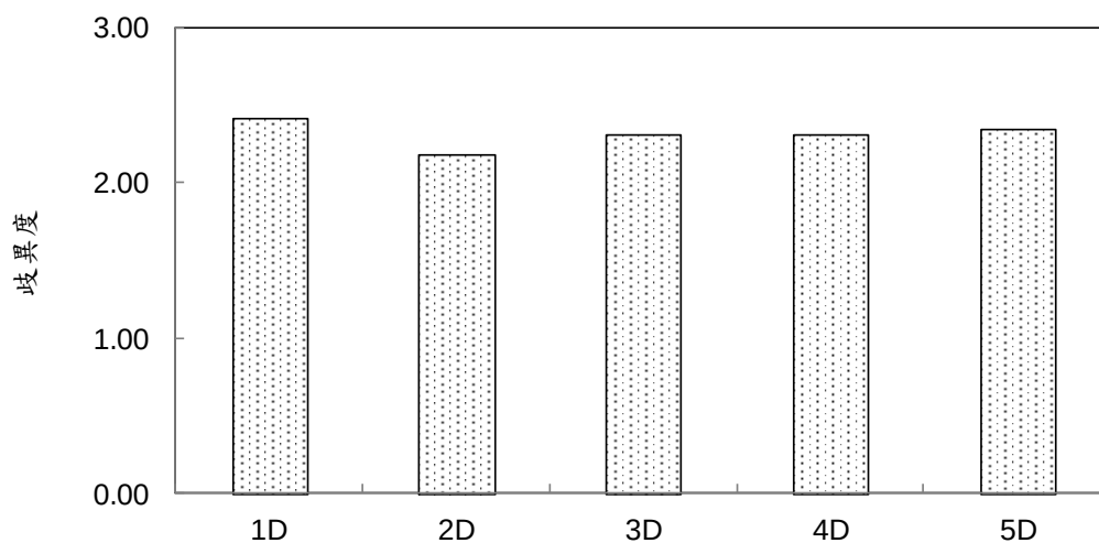
圖 2.9.2-6 110 年第 1 季河口各測站之浮游動物歧異度變化圖
