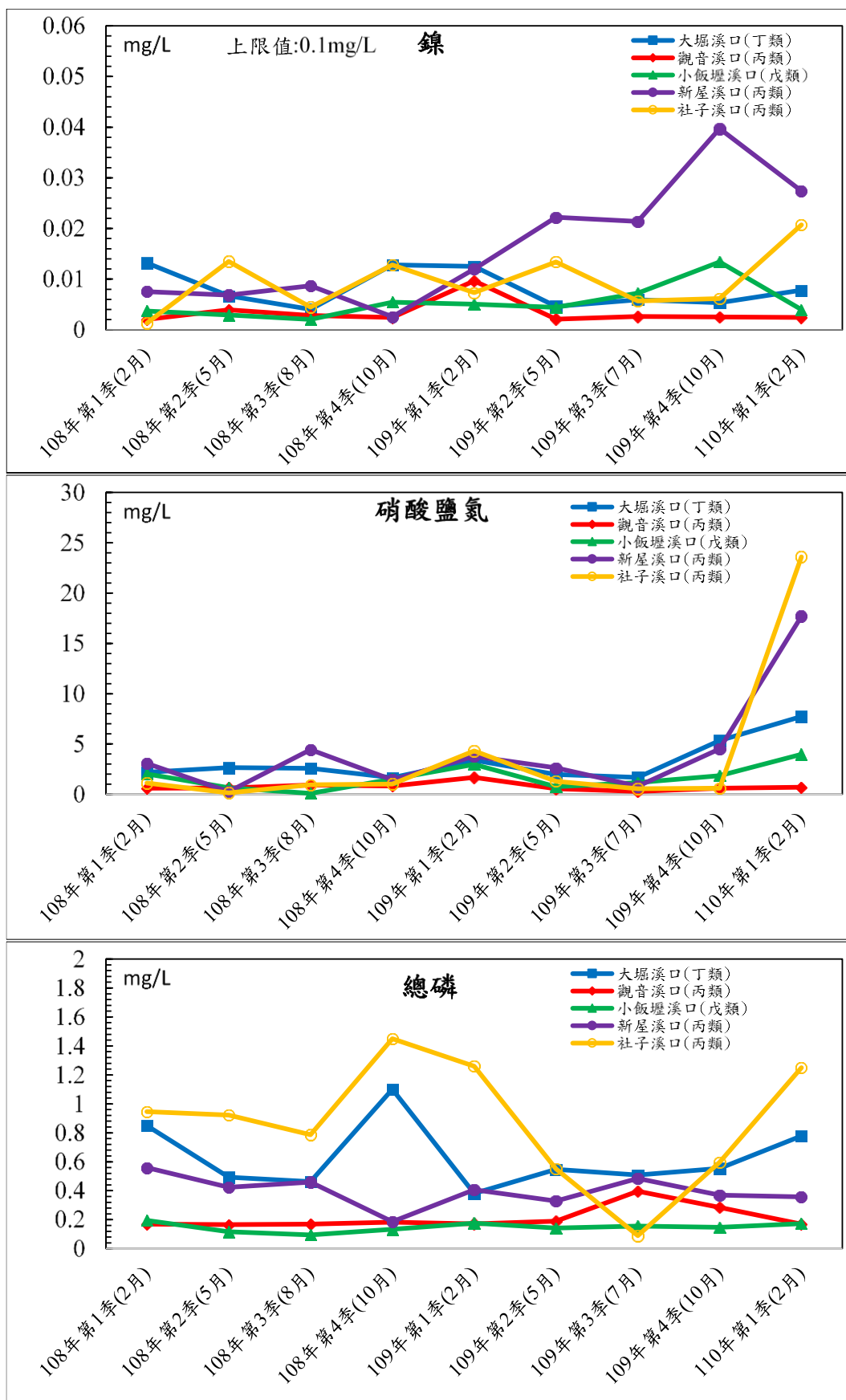
圖 3.1.7-1 歷次河口水質監測結果分析圖(7/8)
