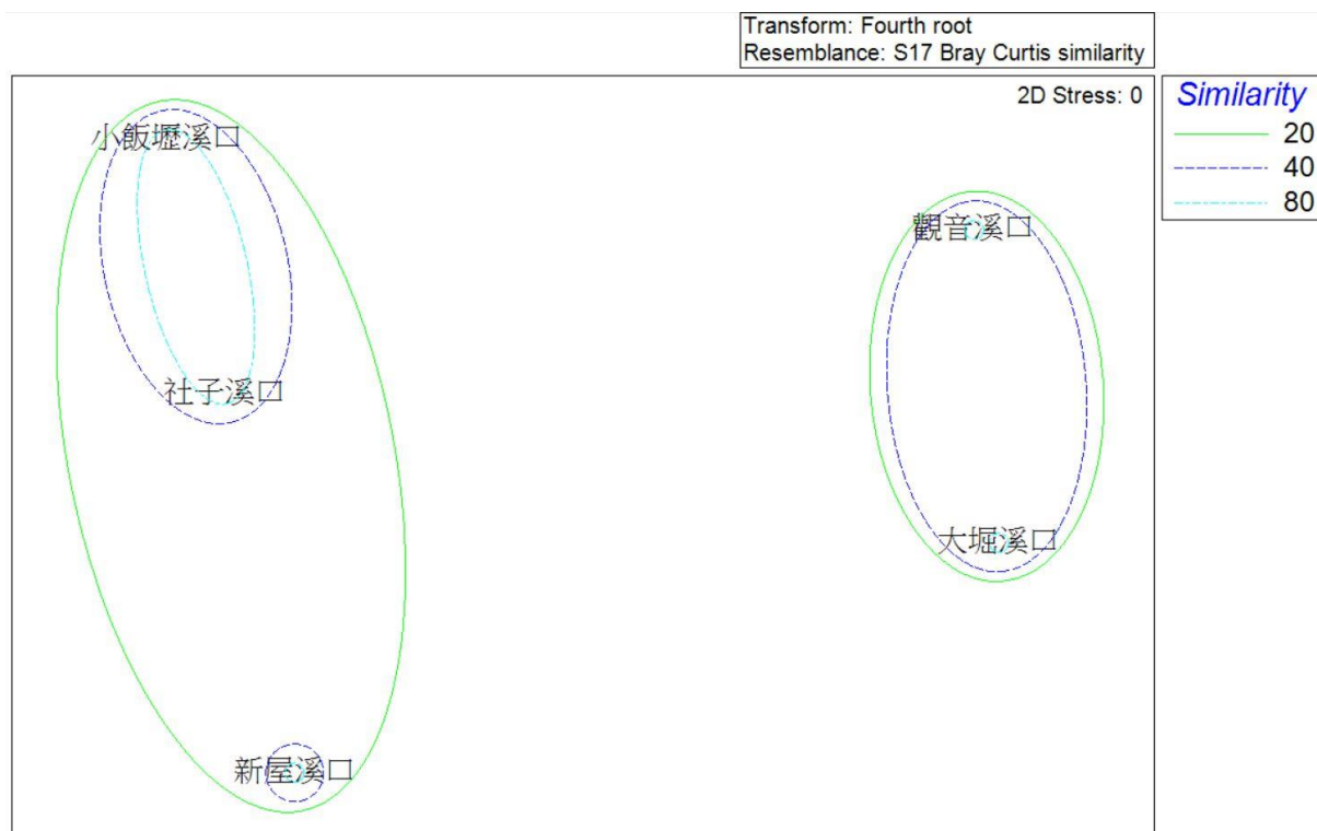
圖 2.9.3-5 110 年第 1 季河口各測站底棲生物之 MDS 圖
