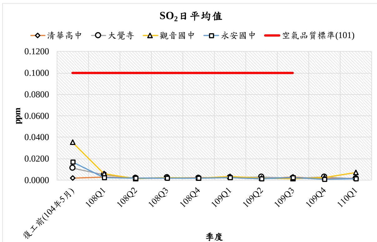
圖 3.1.2-5 SO 2 日平均值監測結果分析圖
