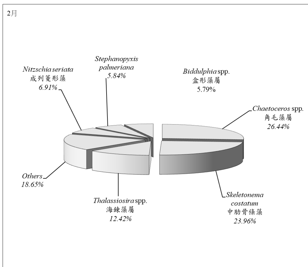
圖 2.8.1-2 110 年第 1 季海域各類浮游植物優勢大類數量百分比
