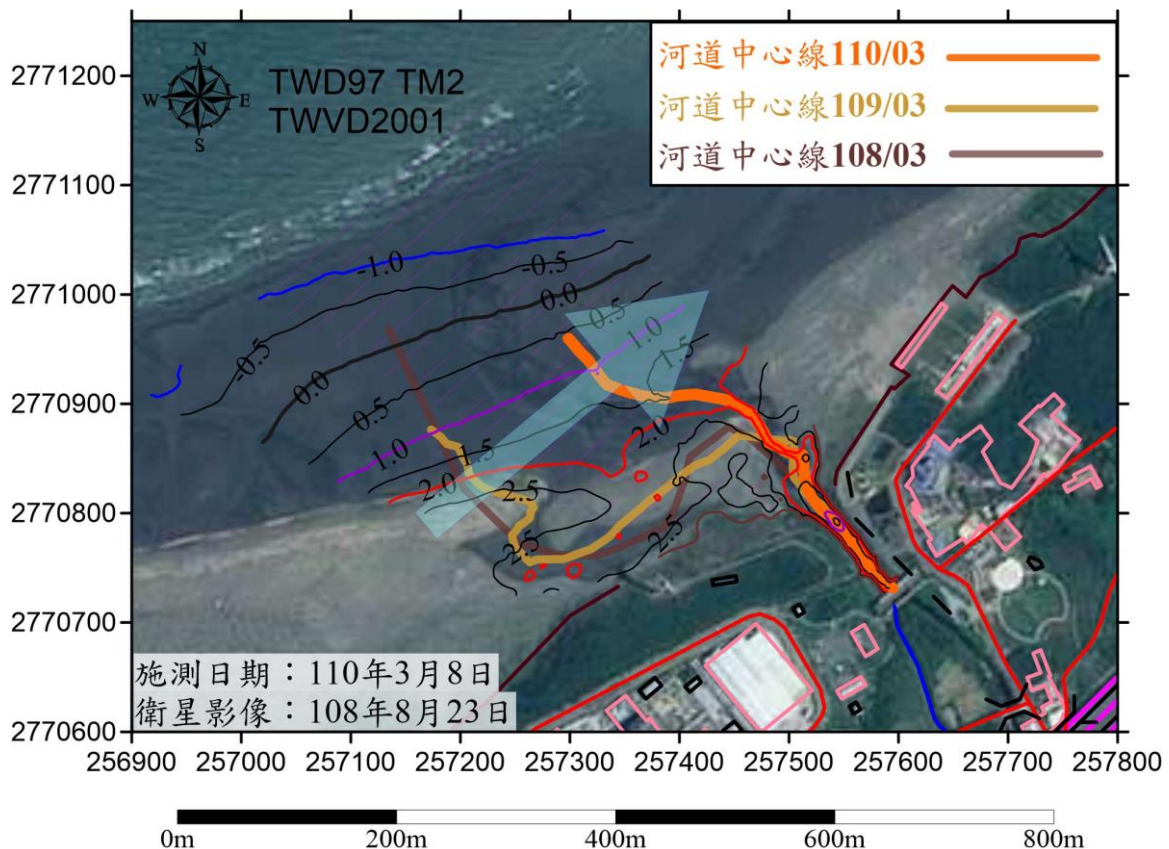
圖 3.1.13.1-1 108 年 3 月至 110 年 3 月觀音溪河道中心線變遷圖
