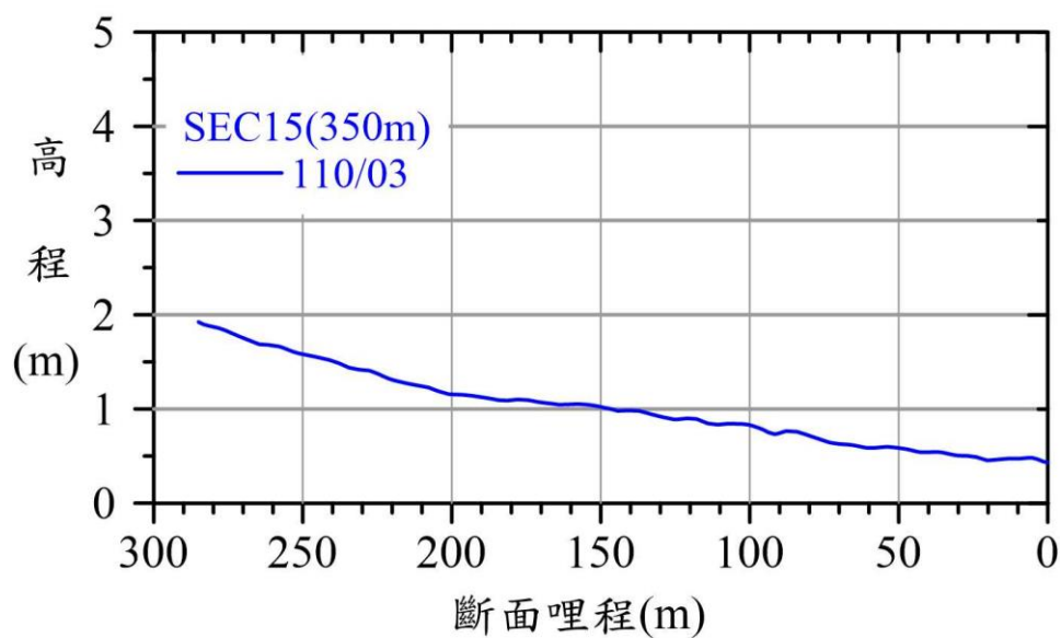
圖 2.12.1-10 觀音溪河口地形斷面圖(SEC13~SEC15)
