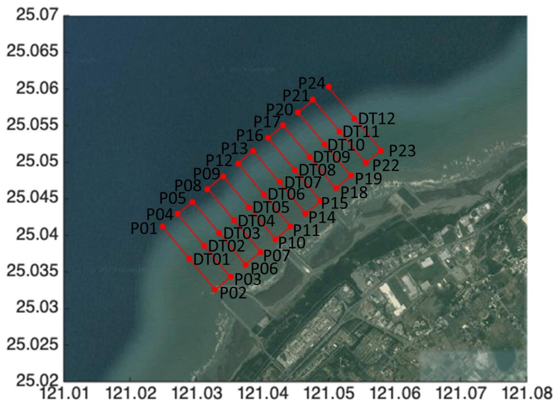
圖 1.8.2-1 原施工海域空間濃度變化監測規劃剖面位置圖
