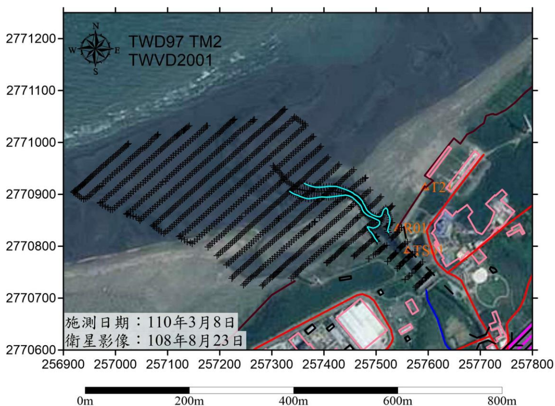
圖 2.12.1-1 110 年 3 月 8 日觀音溪河口地形施測點位圖
