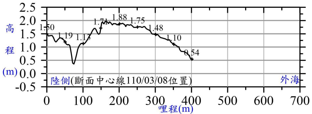
圖 2.12.1-4 觀音溪 110 年河道中心線底床高程剖面圖
