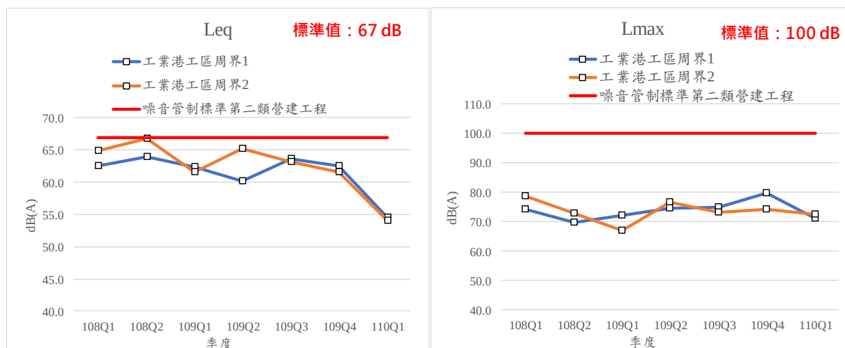
圖 3.1.4-1 歷次營建噪音監測結果分析圖
