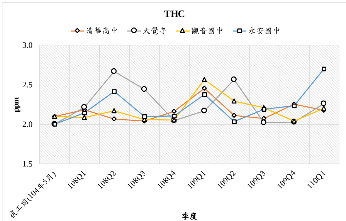
圖 3.1.2-10 THC 監測結果分析圖
