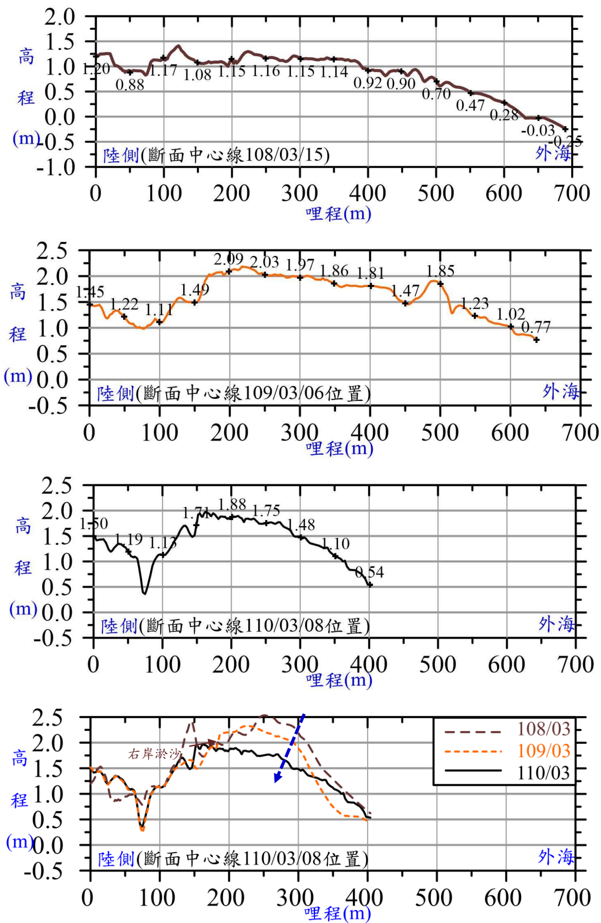
圖 3.1.13.1-2 108 年至 110 年河道中心線底床高程剖面圖
