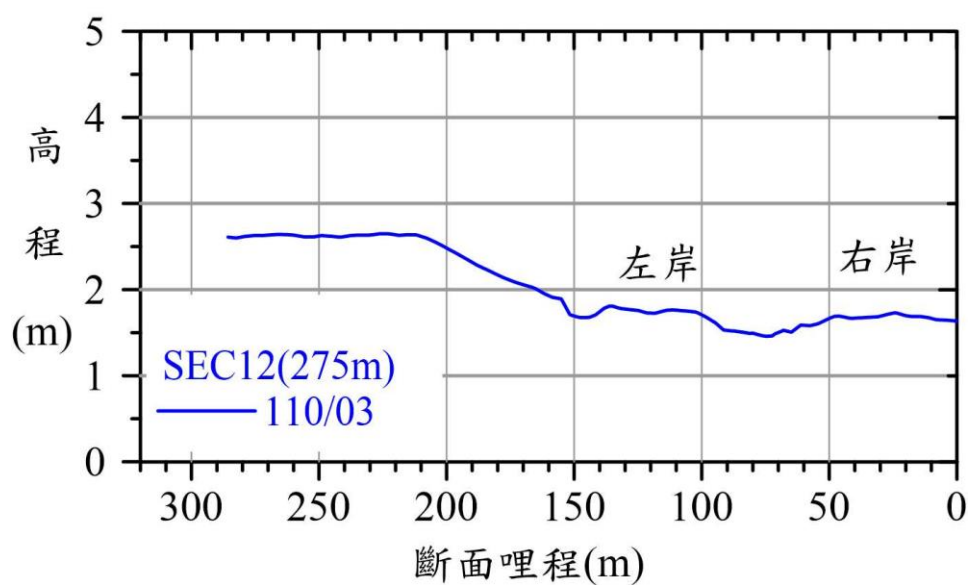
圖 2.12.1-9 觀音溪河口地形斷面圖(SEC010~SEC12)
