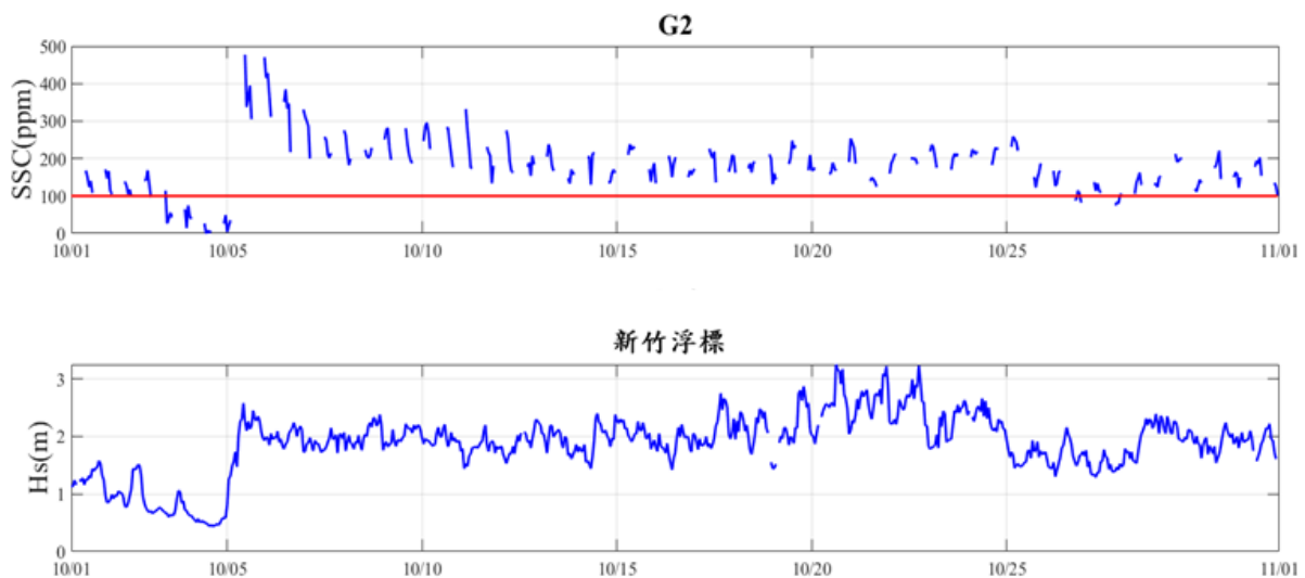
圖 2.11.1-2 本計畫漂沙濃度(109 年 10 月)與新竹浮標波高資料比對圖
