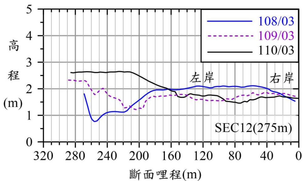
圖 3.1.13.1-6 觀音溪河口地形斷面圖(SEC10~SEC12)
