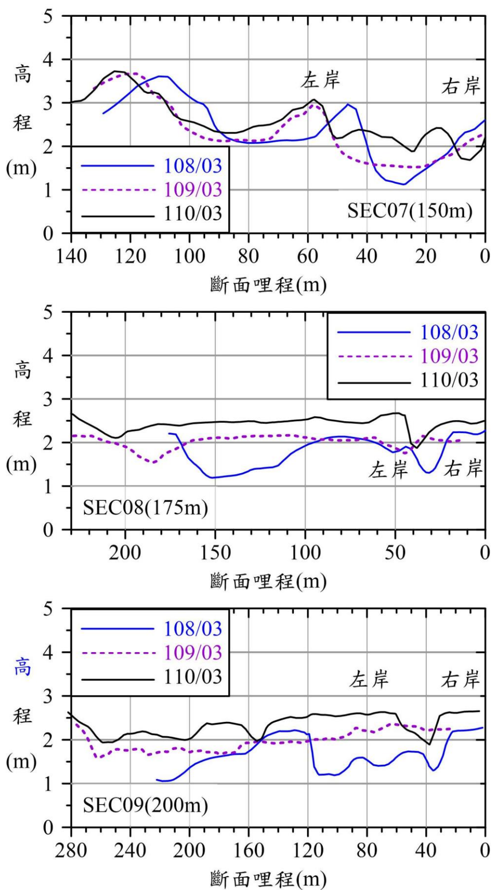
圖 3.1.13.1-5 觀音溪河口地形斷面圖(SEC07~SEC09)
