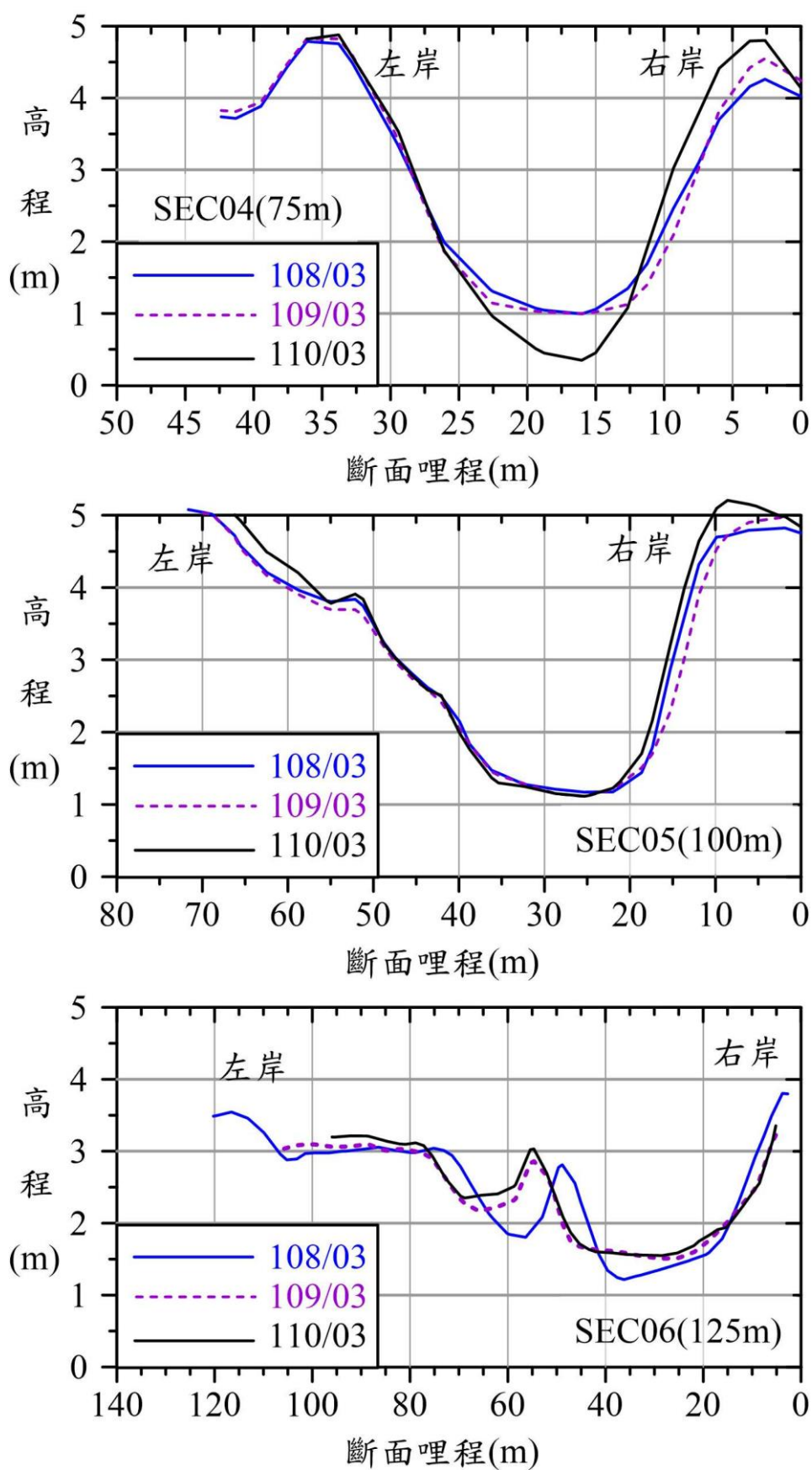
圖 3.1.13.1-4 观音溪河口地形断面图(SEC04~SEC06)
