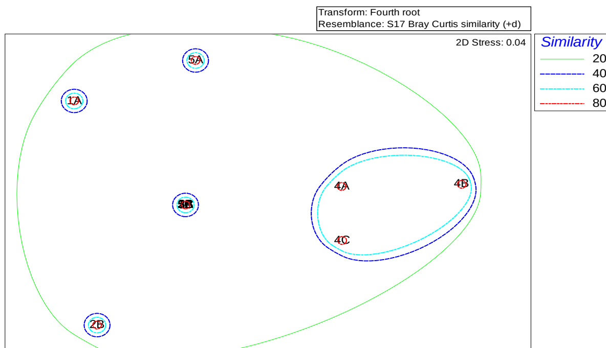
圖 2.8.4-1 110 年第 1 季仔稚魚之群集分析樹狀圖
