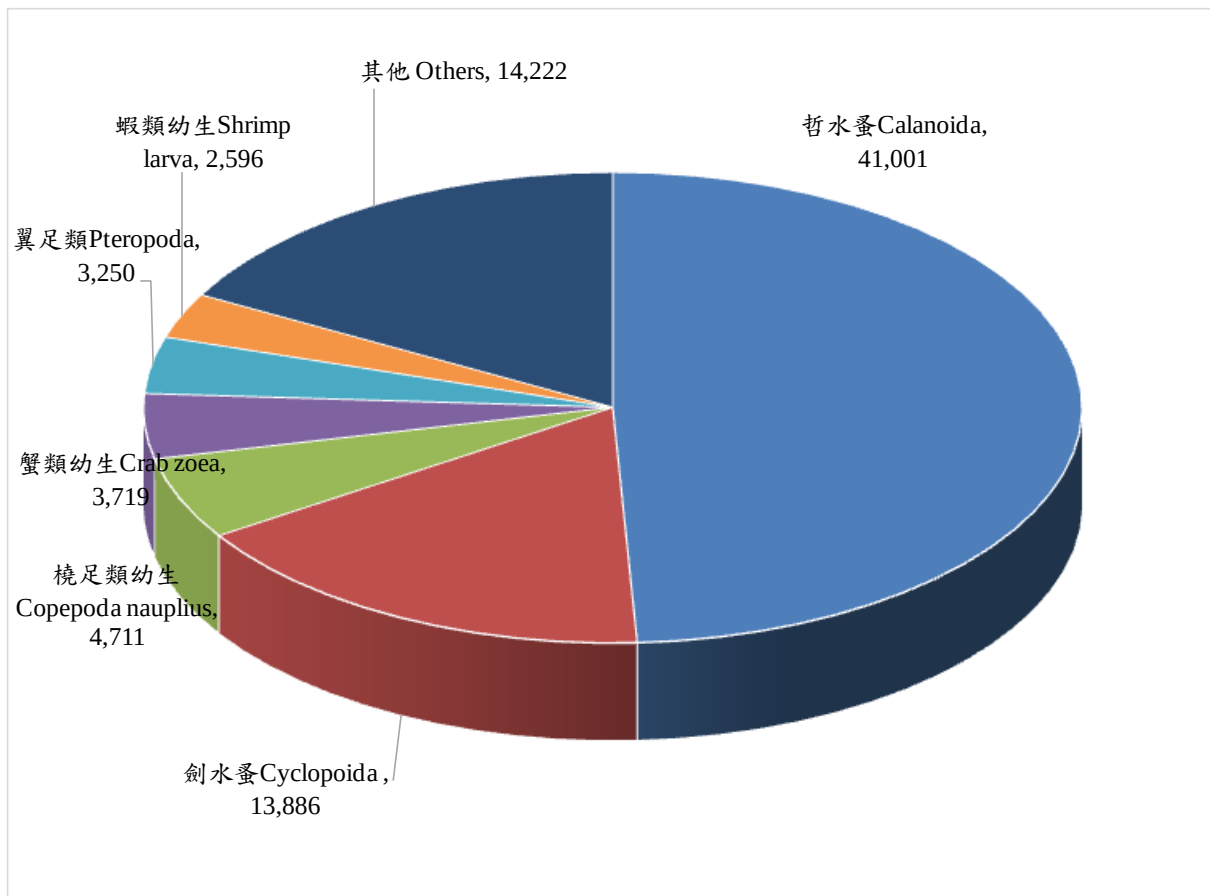
圖 2.8.2-1 110 年第 1 季海域各類浮游動物優勢大類數量百分比
