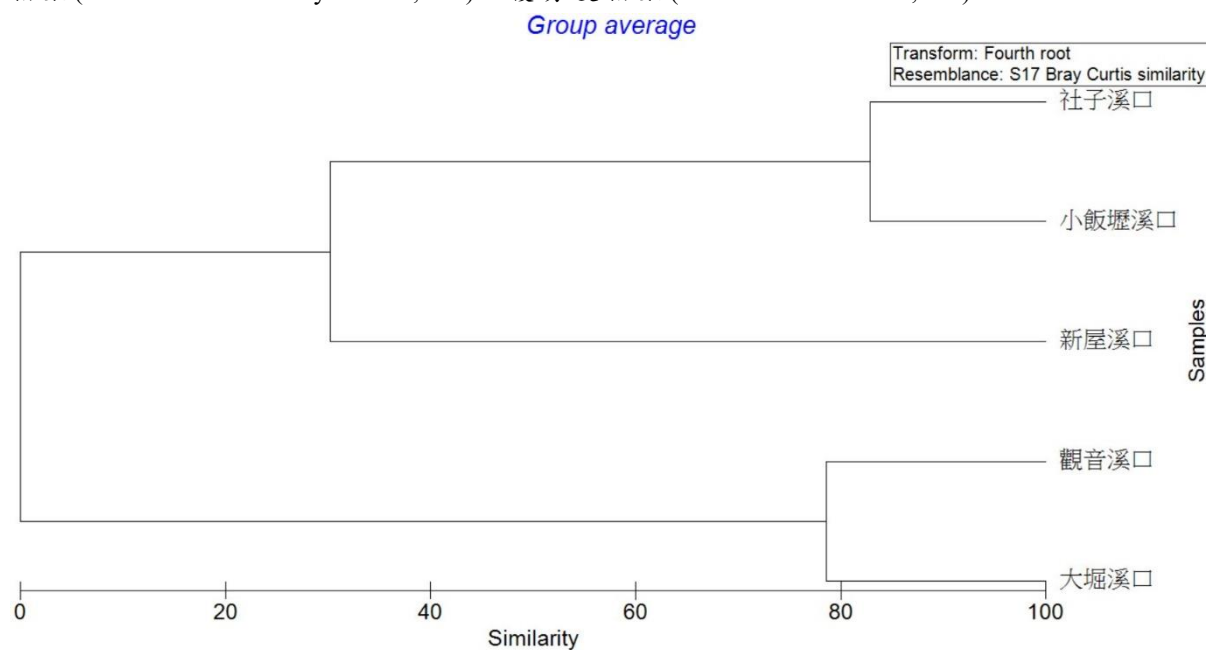
圖 2.9.3-4 110 年第 1 季河口各測站採得底棲生物之群集分析樹狀圖
