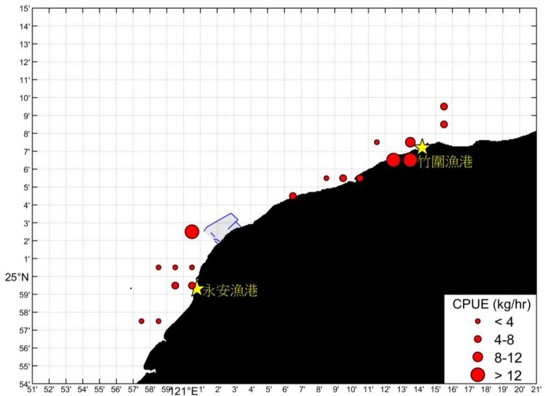
圖 2.10.2-9 110 年 1 月桃園地區每單位努力漁獲量(CPUE)分布
