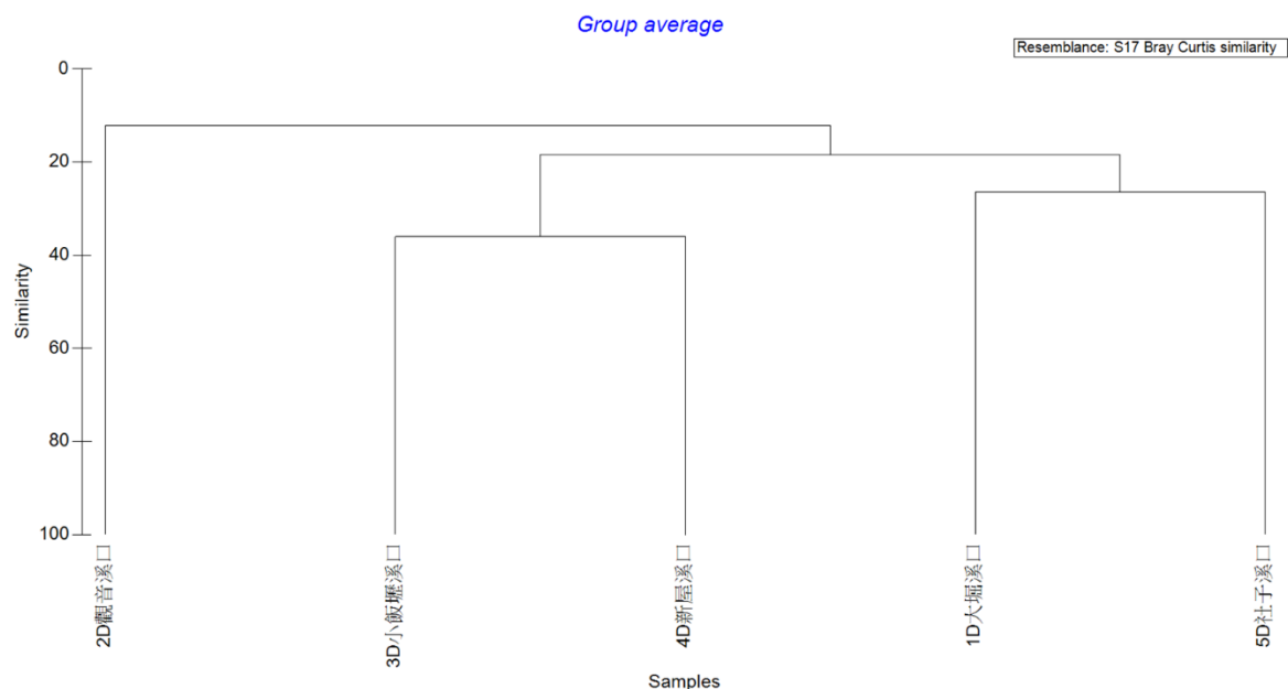
圖 2.9.1-3 110 年第 1 季河口各測站之浮游植物之群集分析圖
