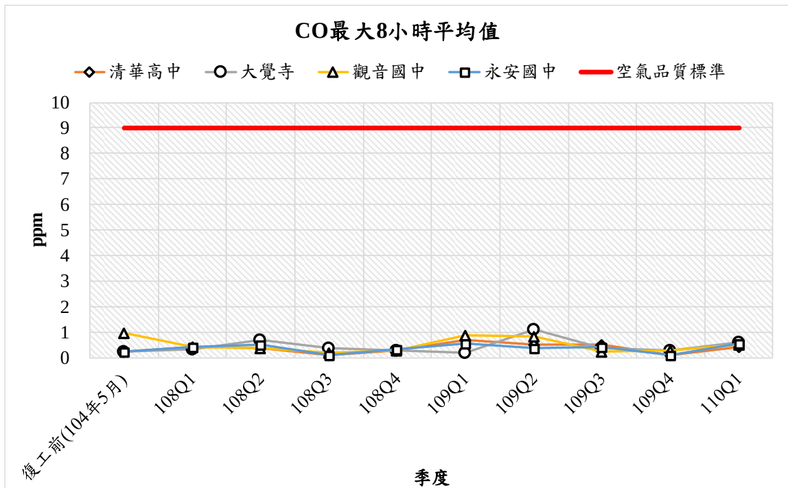
圖 3.1.2-9 CO 最大 8 小時平均值監測結果分析圖
