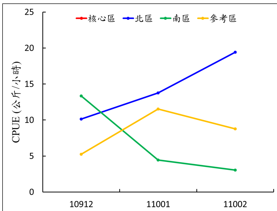
圖 2.10.2-13 110 年第 1 季分區海域月別 CPUE
