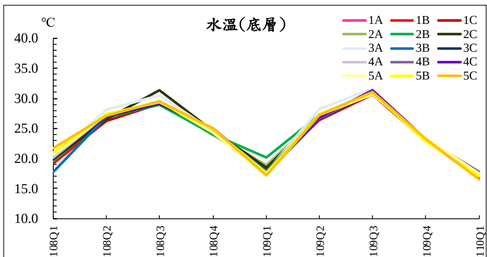
圖 3.1.8-1 歷次海域水質監測結果分析圖(1/17)
