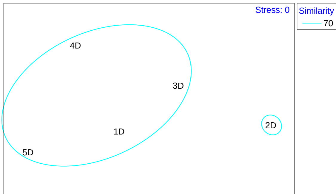
圖 2.9.2-9 110 年第 1 季河口各測站之浮游動物群集分析圖
