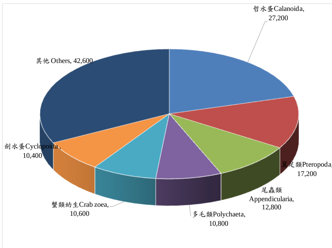
圖 2.9.2-1 110 年第 1 季河口浮游動物優勢大類數量百分比
