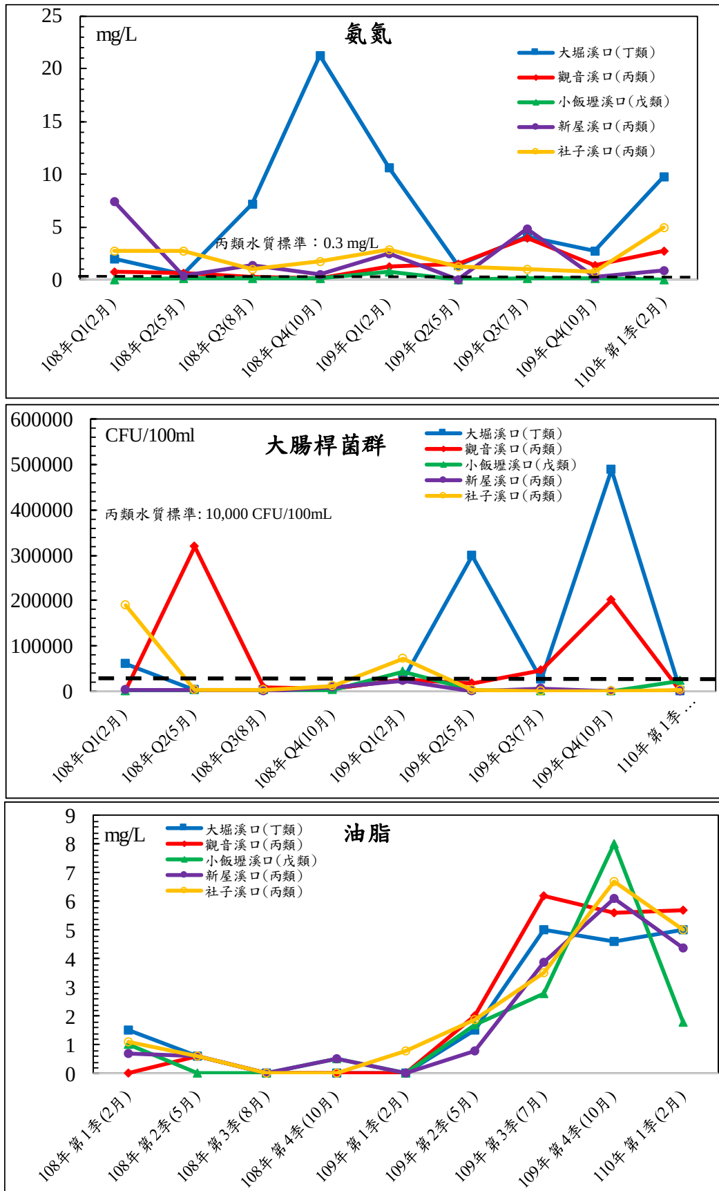
圖 3.1.7-1 歷次河口水質監測結果分析圖(3/8)
