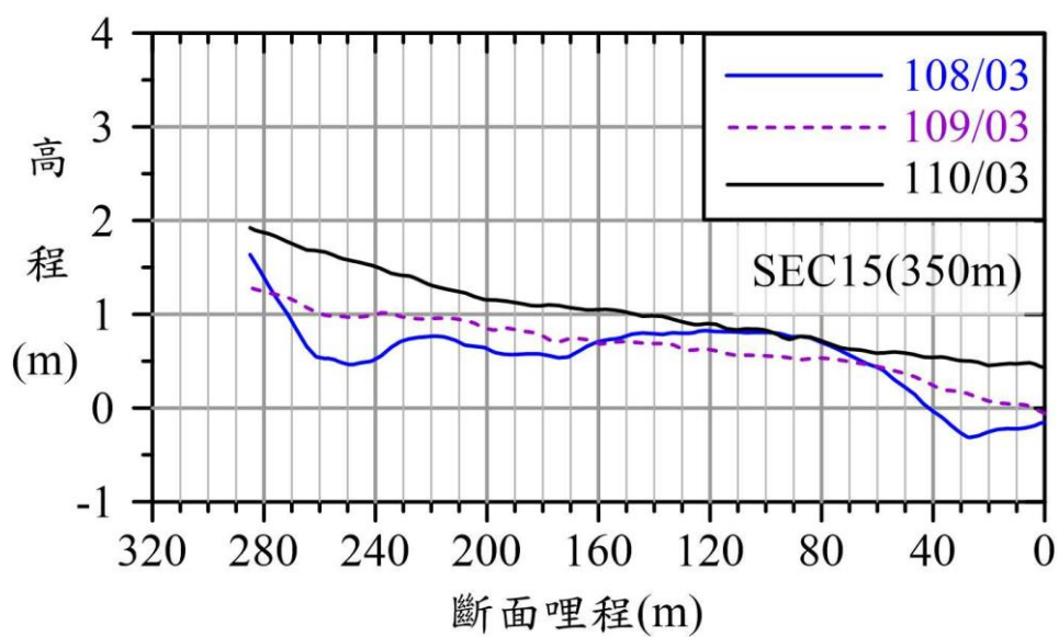
圖 3.1.13.1-7 觀音溪河口地形斷面圖(SEC13~SEC15)
