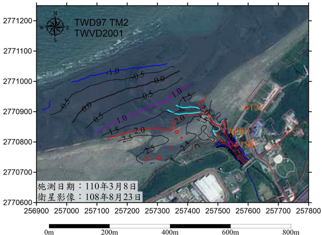
圖 2.12.1-2 110 年 3 月 8 日觀音溪斷面地形施測地形成果圖
