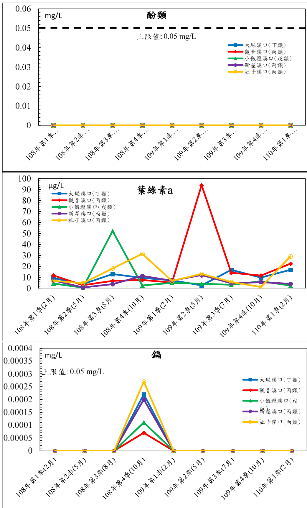
圖 3.1.7-1 歷次河口水質監測結果分析圖(4/8)
