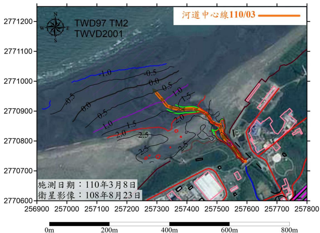
圖 2.12.1-3 110 年 3 月觀音溪河道中心線圖
