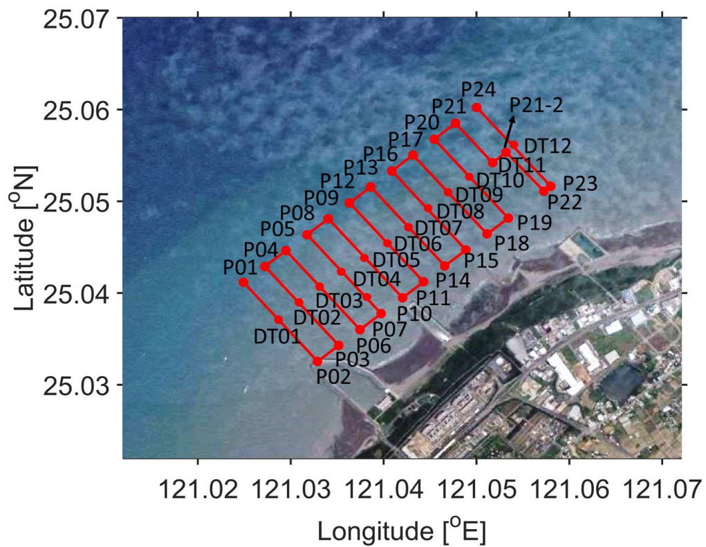
圖 1.8.2-3 本次施工海域空間濃度變化監測規劃剖面位置圖
