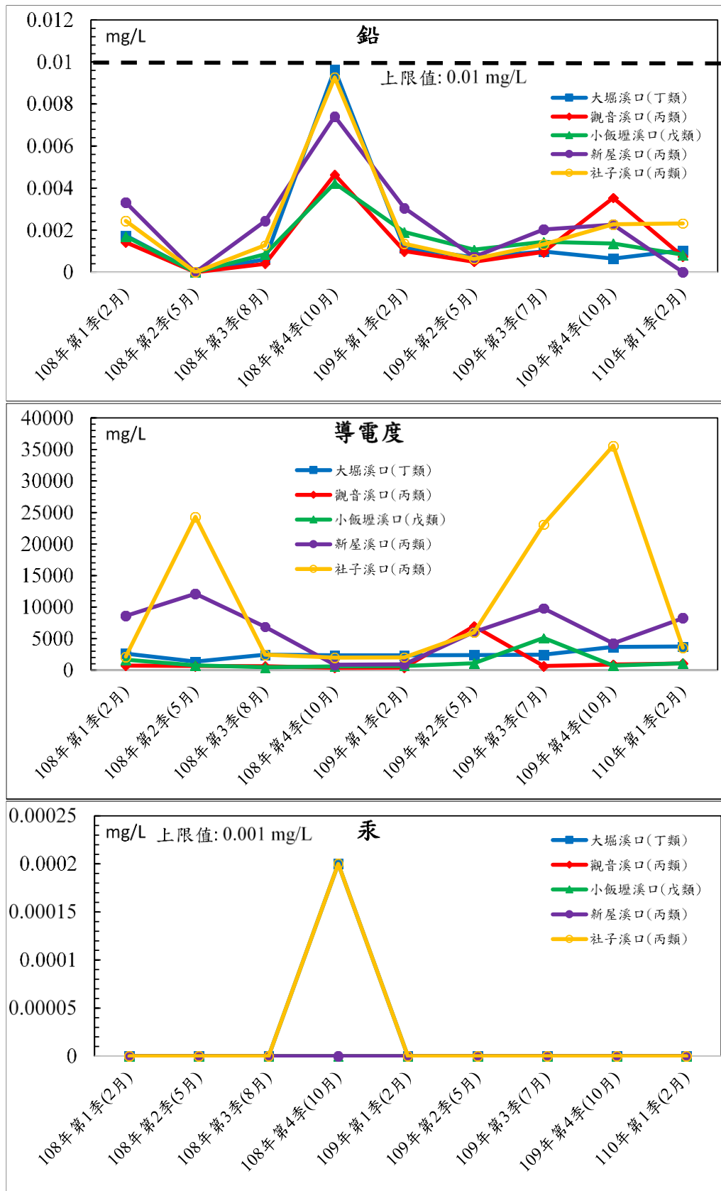
圖 3.1.7-1 歷次河口水質監測結果分析圖(5/8)
