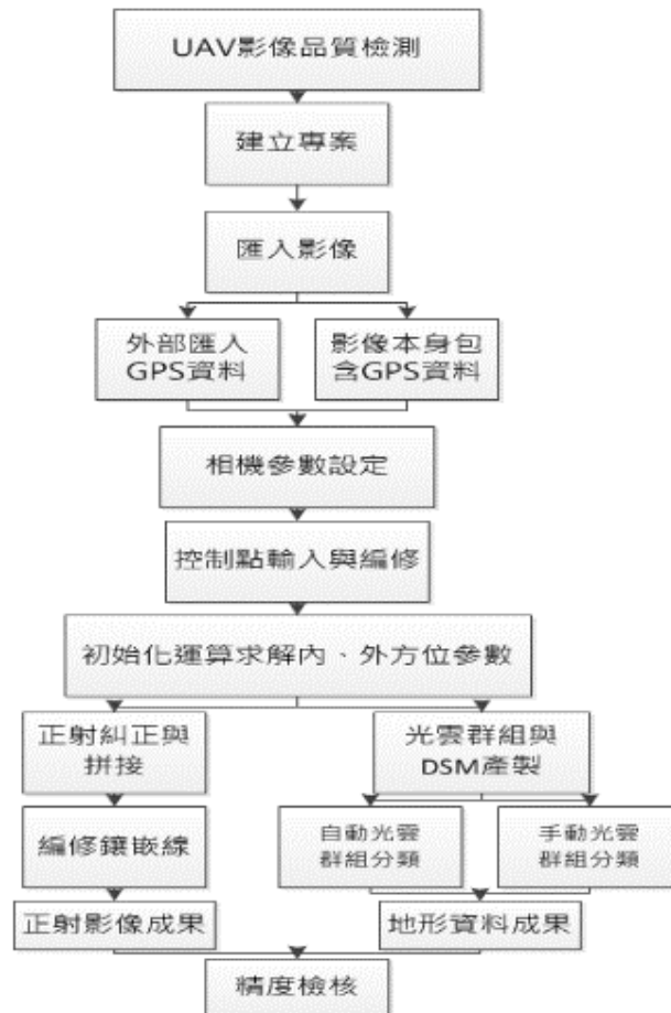
圖 1.10.1-4 Pix4Dmapper 處理軟體作業流程圖
