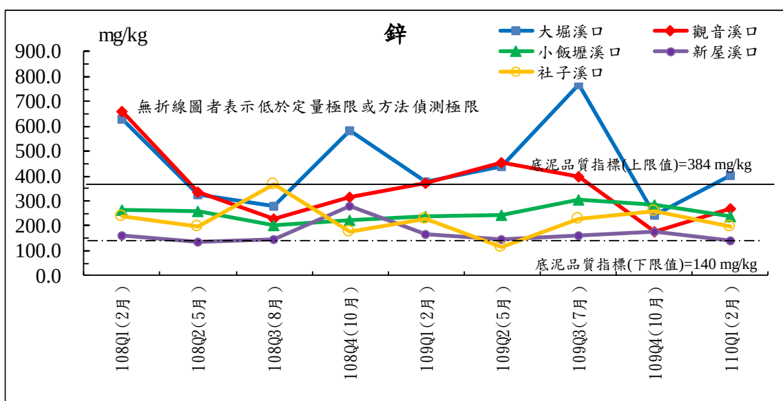
圖 3.1.7-2 歷次河口底泥監測結果分析圖(1/3)
