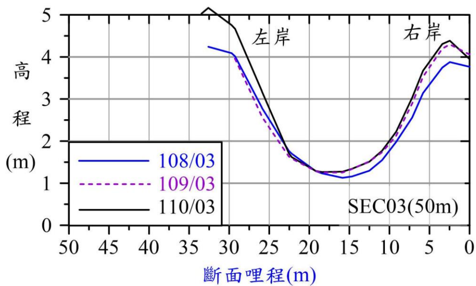
圖 3.1.13.1-3 觀音溪河口地形斷面圖(SEC01~SEC03)
