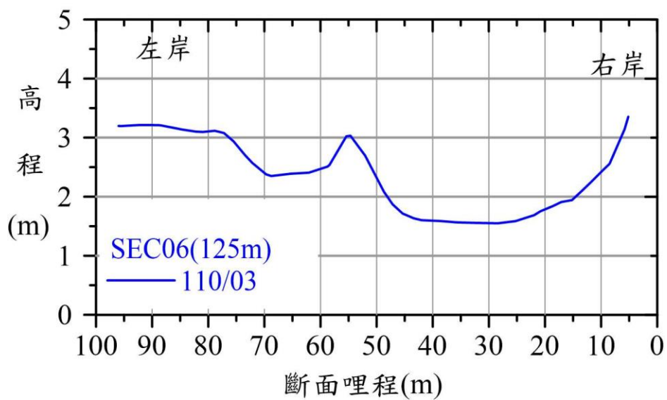
圖 2.12.1-7 觀音溪河口地形斷面圖(SEC04~SEC06)
