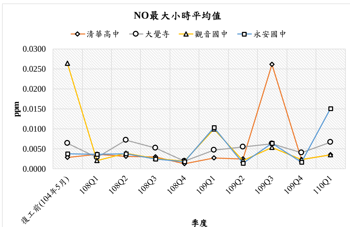
圖 3.1.2-6 NO 最大小時平均值監測結果分析圖
