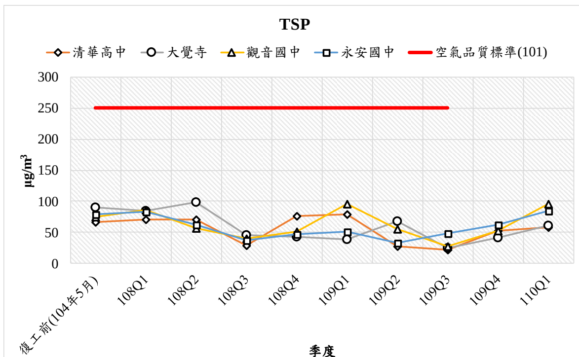
圖 3.1.2-1 TSP 監測結果分析圖
