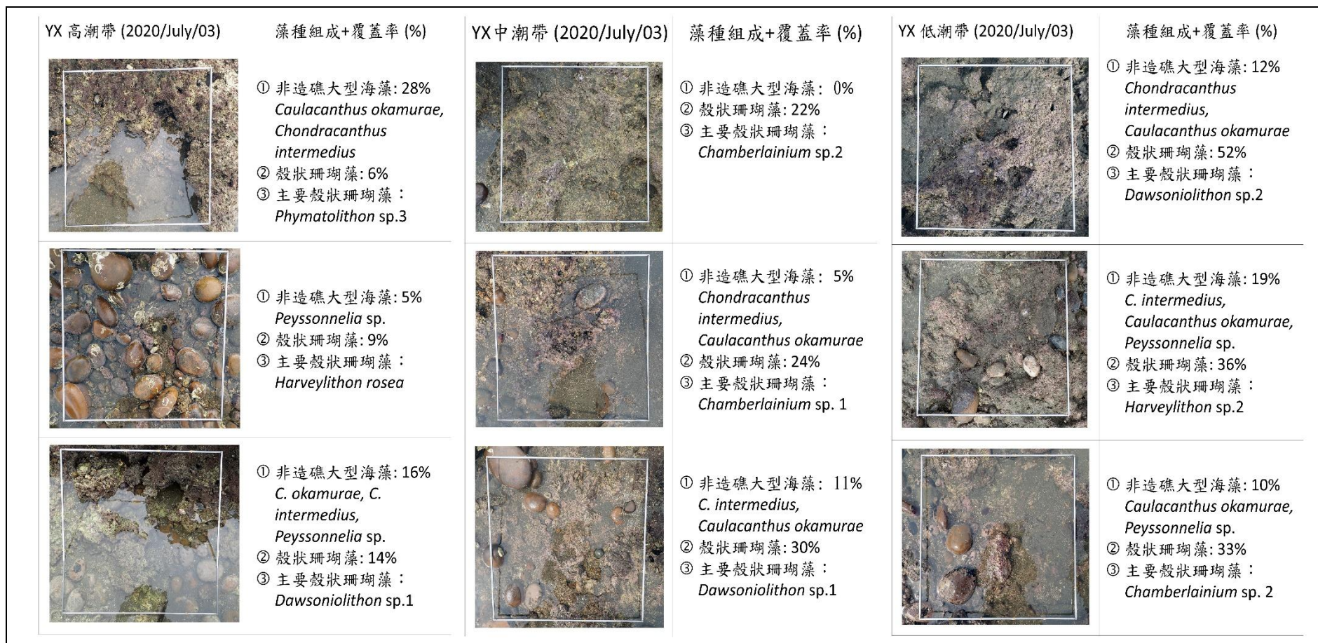
圖 8：109 年 7 月觀新藻礁區測站 2（永興）的殼狀珊瑚藻及大型藻類的藻種組成及覆蓋率。
