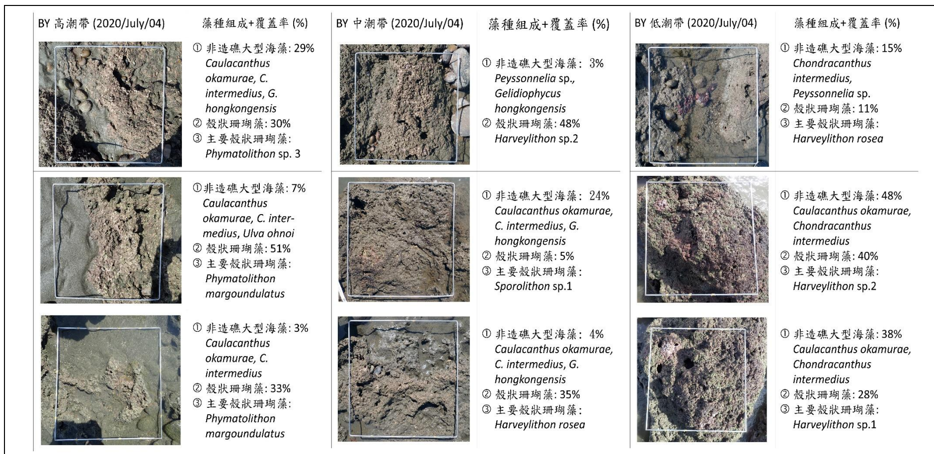
圖 12： 109 年 7 月白玉藻礁區測站 6（白玉）的殼狀珊瑚藻及大型藻類的藻種組成及覆蓋率。
