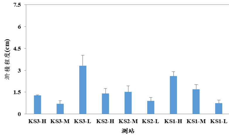
圖 12：109 年 3 月各測站淤積程度結果
