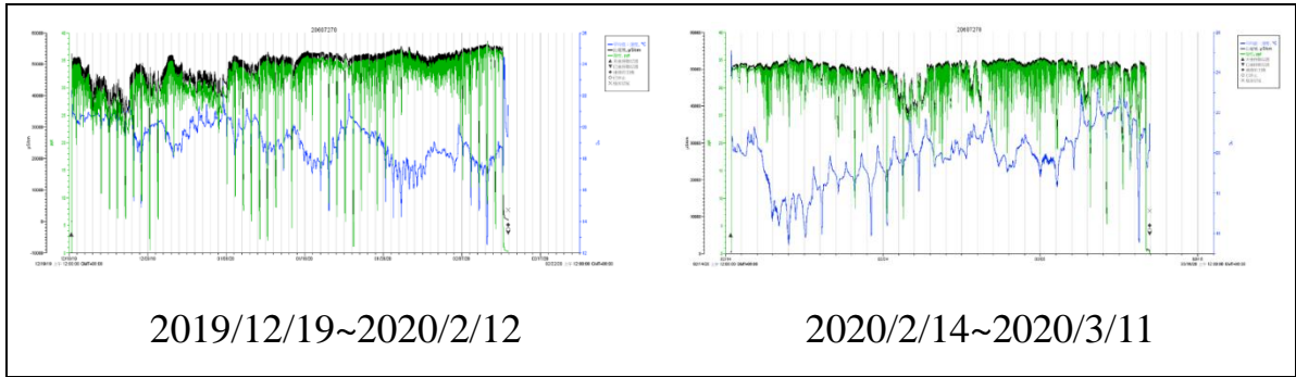
圖 6：白玉區水溫鹽度長期監測資料（藍:水溫，綠:鹽度）
