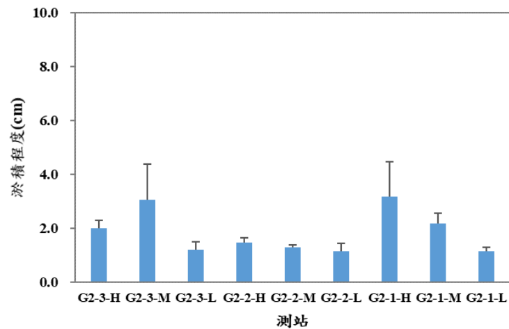
圖 10：109 年 1 月各測站淤積程度結果
