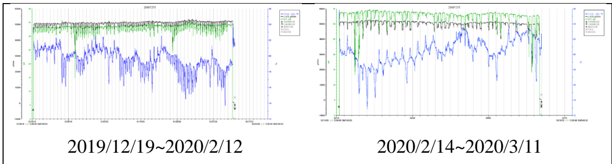
圖 7：觀新區水溫鹽度長期監測資料（藍:水溫，綠:鹽度）
