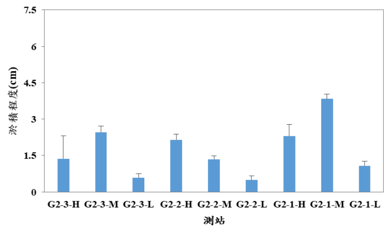
圖 11：109 年 2 月各測站淤積程度結果
