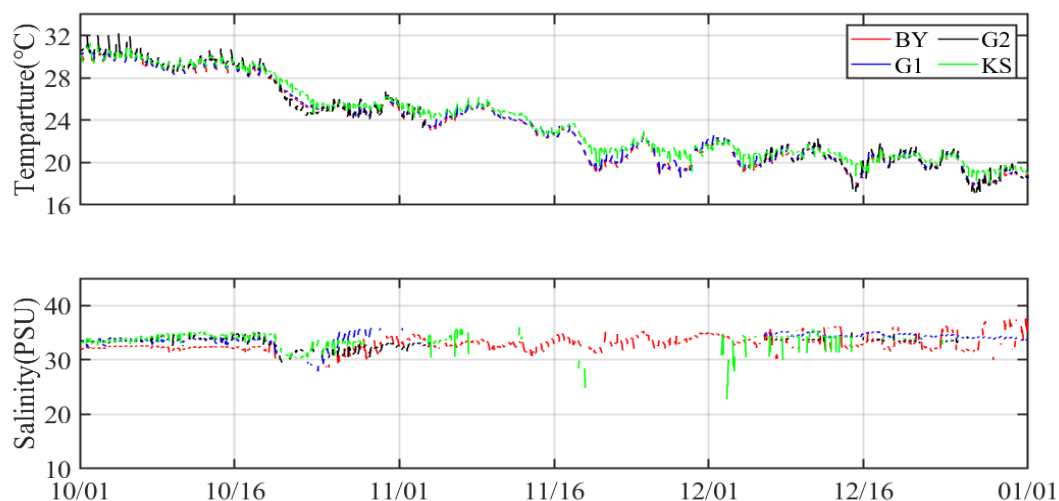
圖 6、114 年第 4 季 (10-12 月) 水溫與鹽度監測資料
