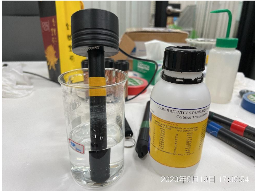
圖 2、導電度探頭校正工作照
