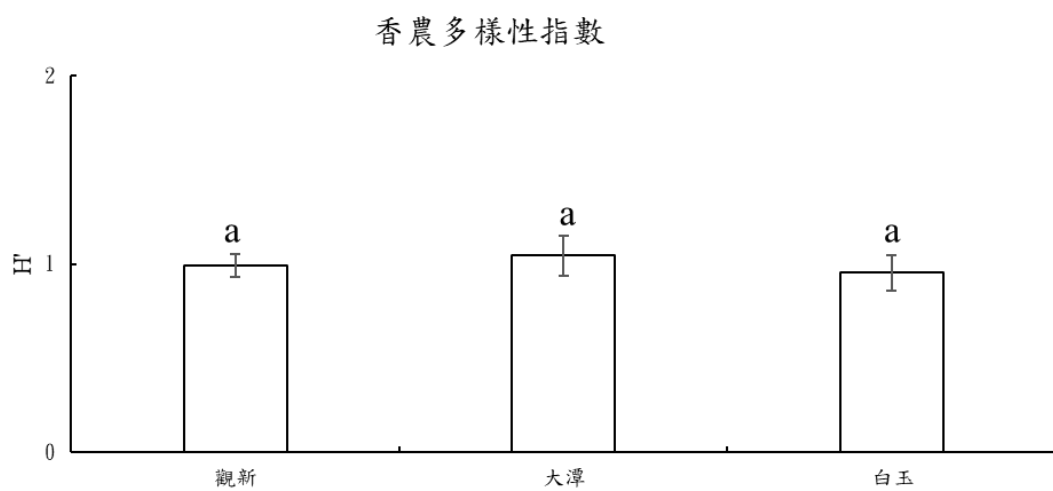
圖 4、113 年第 4 季各調查樣區之物種數、豐度及香農多樣性指數
