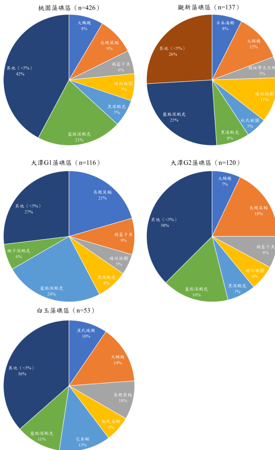
圖 2、113 年第 4 季調查研究樣區魚種組成。
