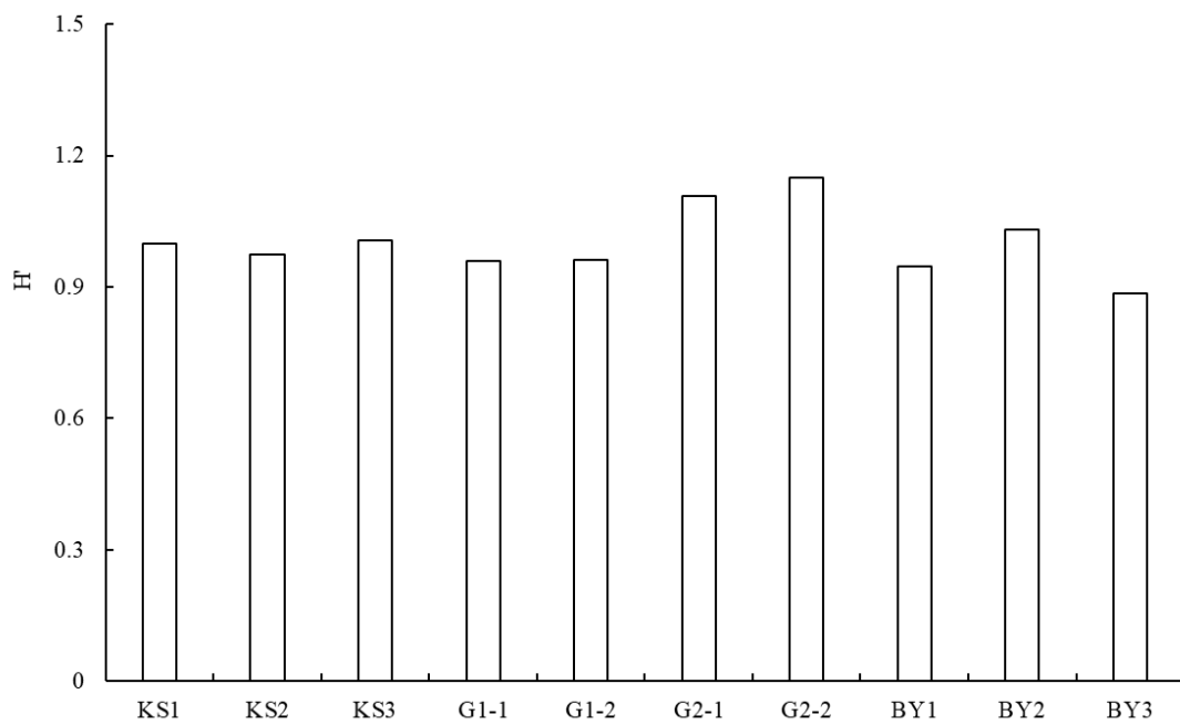
圖 3、113 年第 4 季各調查測站之物種數、豐度及香農多樣性指數
