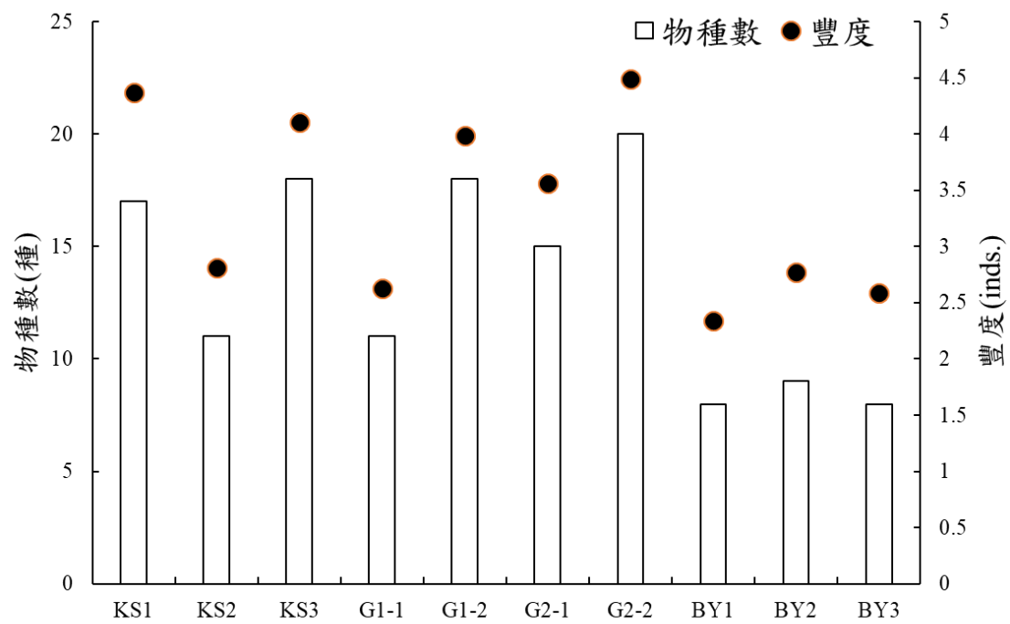
香農多樣性指數
