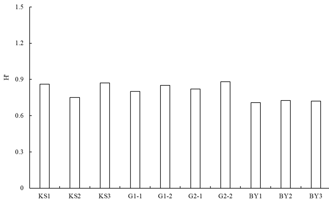
圖 3、113 年第 2 季各調查測站之物種數、豐度及香農多樣性指數
