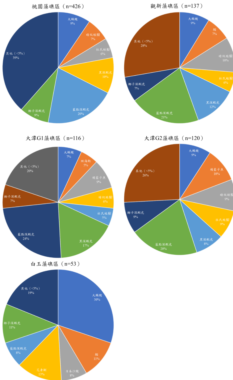
圖 2、113 年第 2 季調查研究樣區魚種組成。
