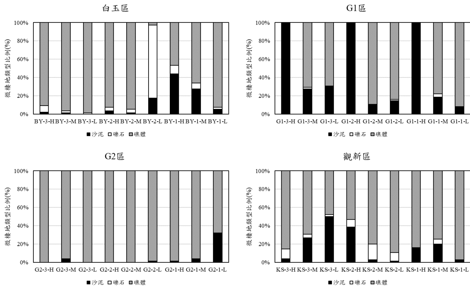
圖 11、113 年第 2 季各測站微棲地底質類型組成比例
