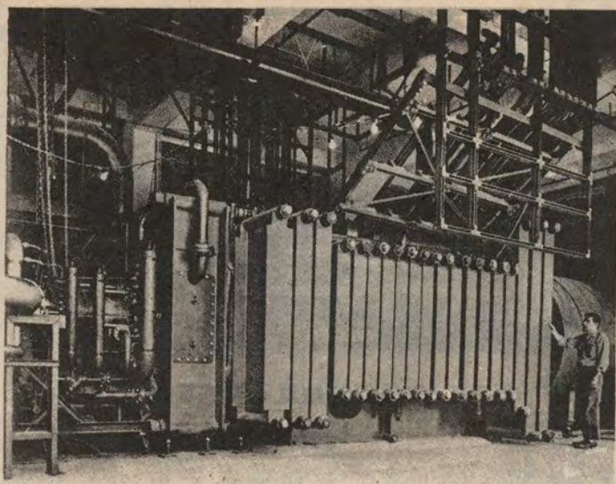
1965 年 AVCO 研究室建造的 Mark V 式 MHD 發電機
