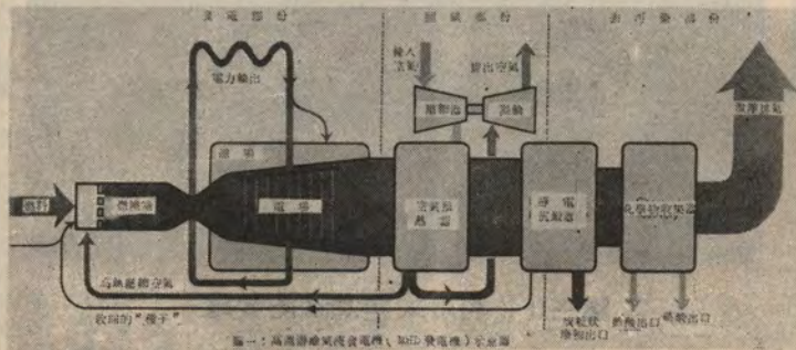
圖一：高溫游離氣流發電機（MHD發電機）示意圖
