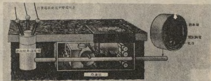
圖二：無損耗的輸電電纜示意圖
